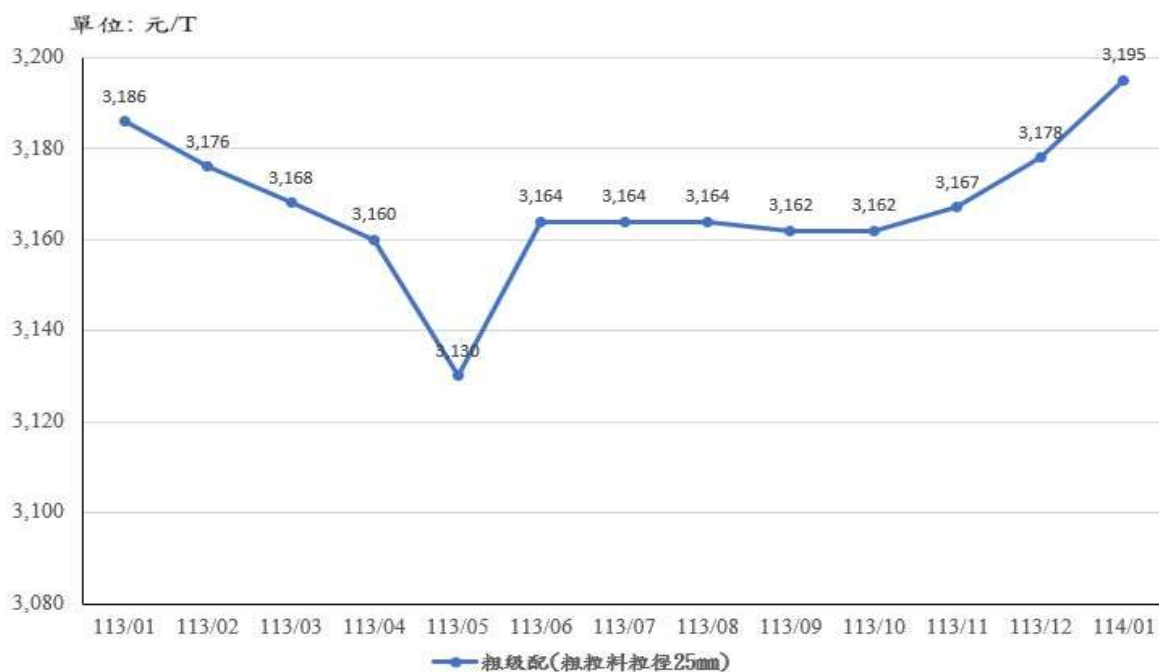
圖 14：113 年 1 月至 114 年 1 月粗級配(粗粒料粒徑 25mm)
