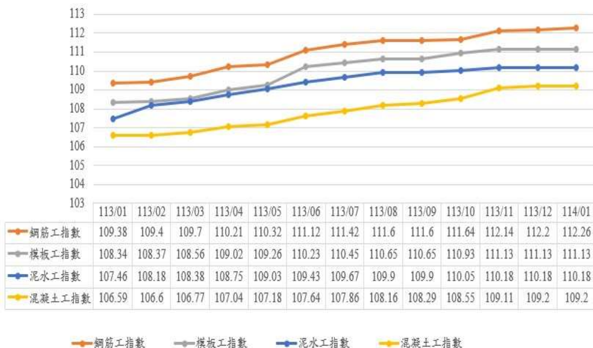
圖 7：113 年 1 月至 114 年 1 月泥水工、鋼筋工、模板工及混凝土工指數走勢
