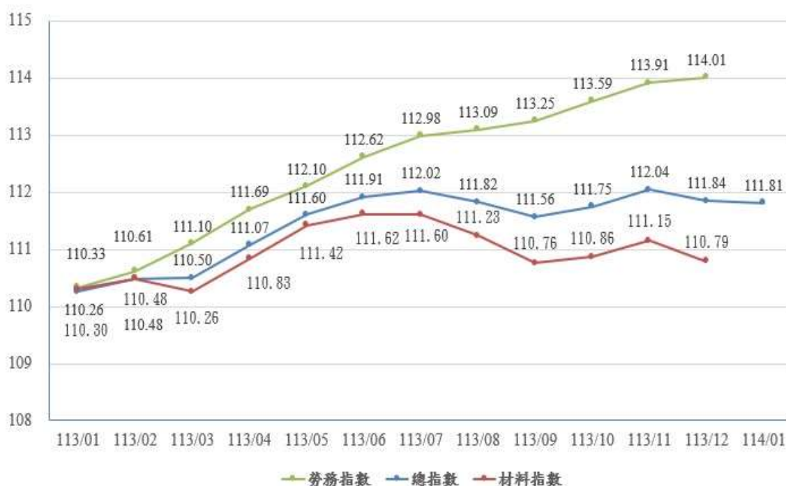
圖 1：113 年 1 月至 114 年 1 月營造工程物價指數走勢；114 年 1 月勞務及材料指數尚未公告。
