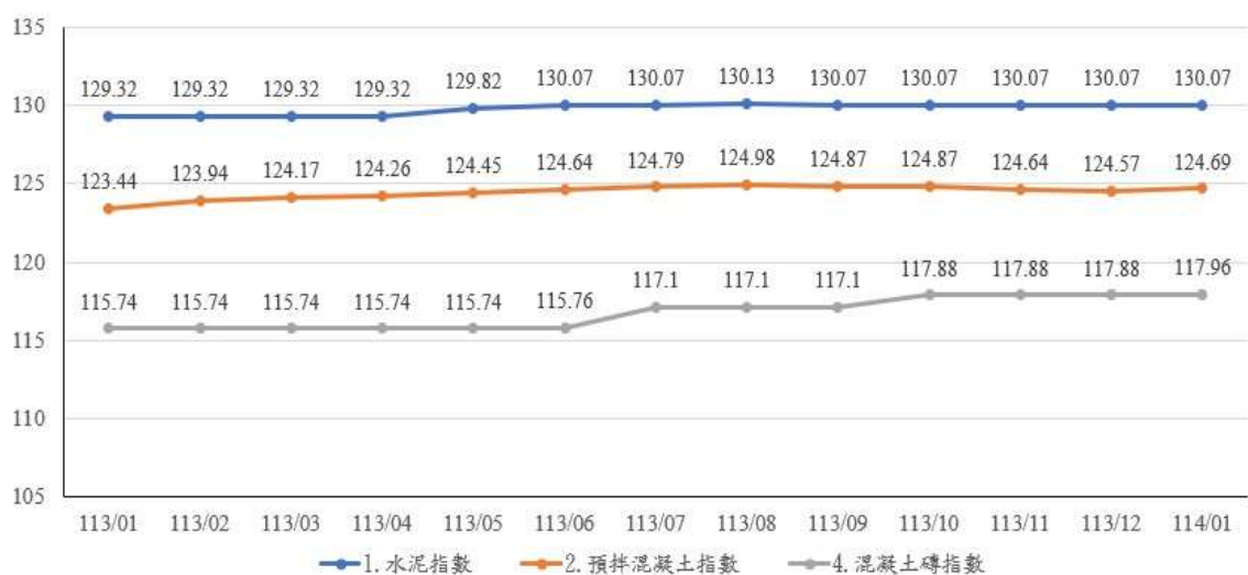
圖 2：113 年 1 月至 114 年 1 月水泥、預拌混凝土及混凝土磚指數走勢
