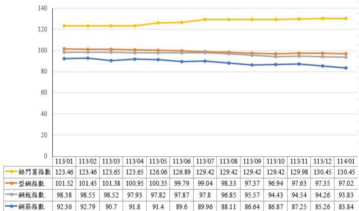
圖 4：113 年 1 月至 114 年 1 月鋼筋、型鋼、鋼板及鋁門窗指數走勢
