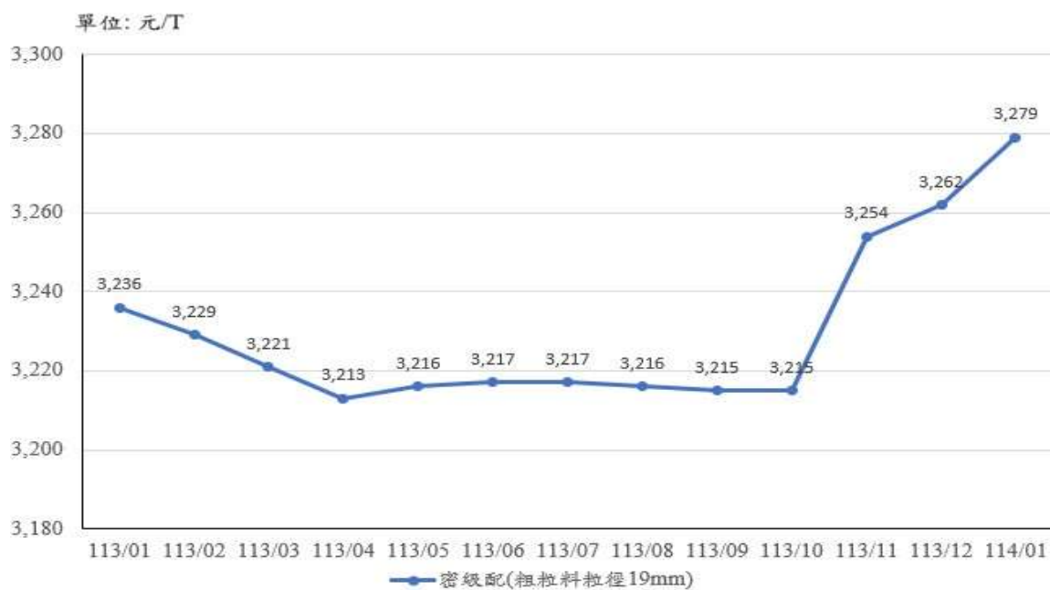
圖 15：113 年 1 月至 114 年 1 月密級配(粗粒料粒徑 19mm)
