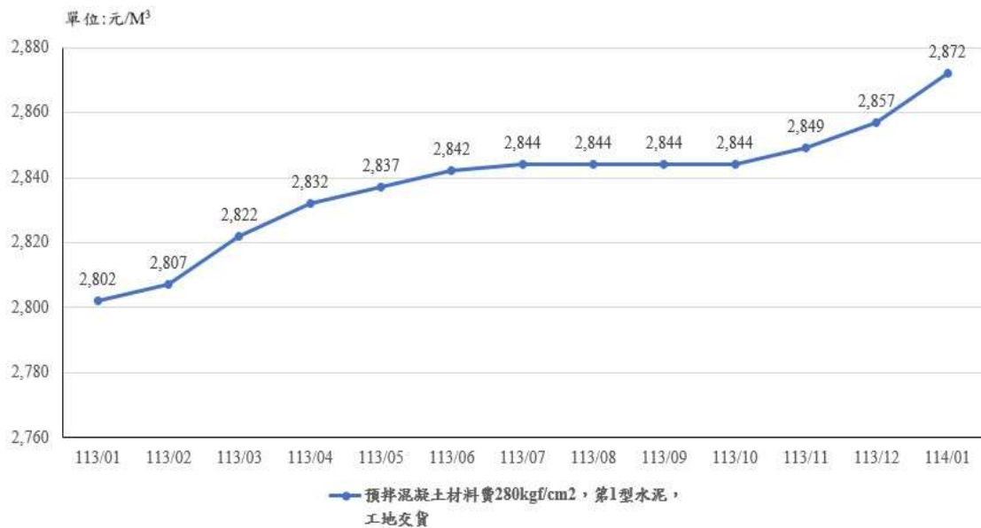
圖 9：113 年 1 月至 114 年 1 月「280kgf/cm 2 ，第 1 型水泥」價格走勢
