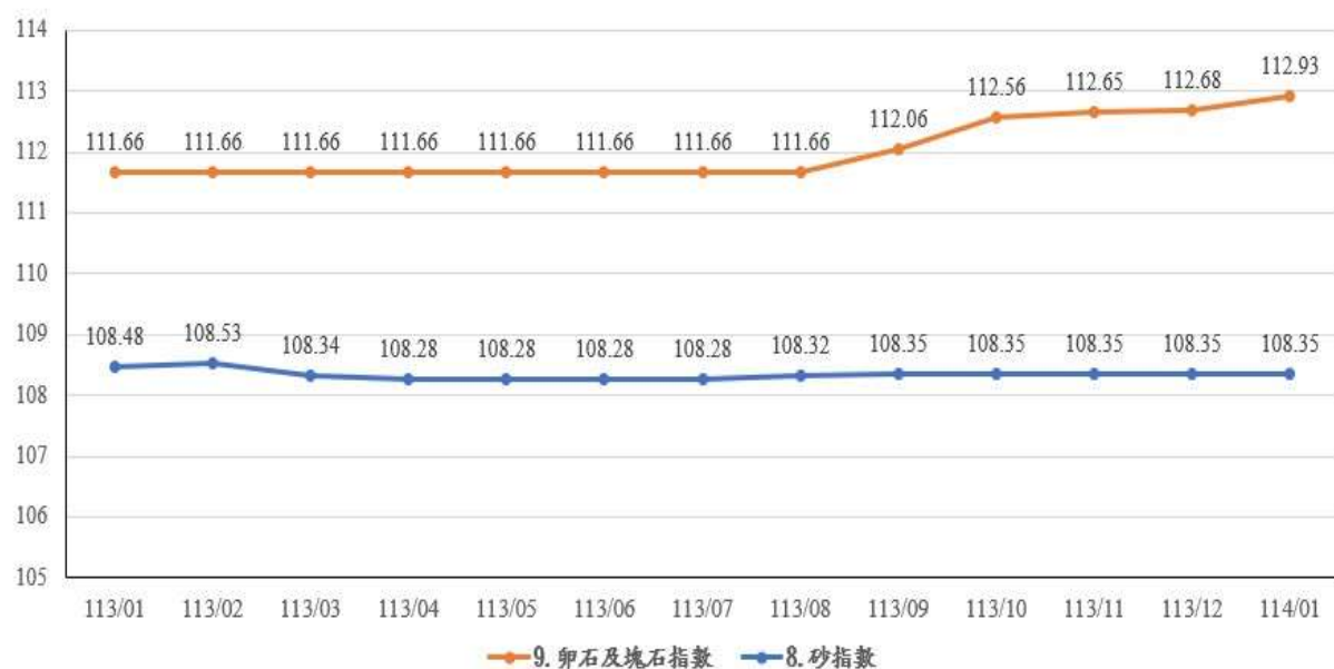
圖 3：113 年 1 月至 114 年 1 月砂、卵石及塊石指數走勢
