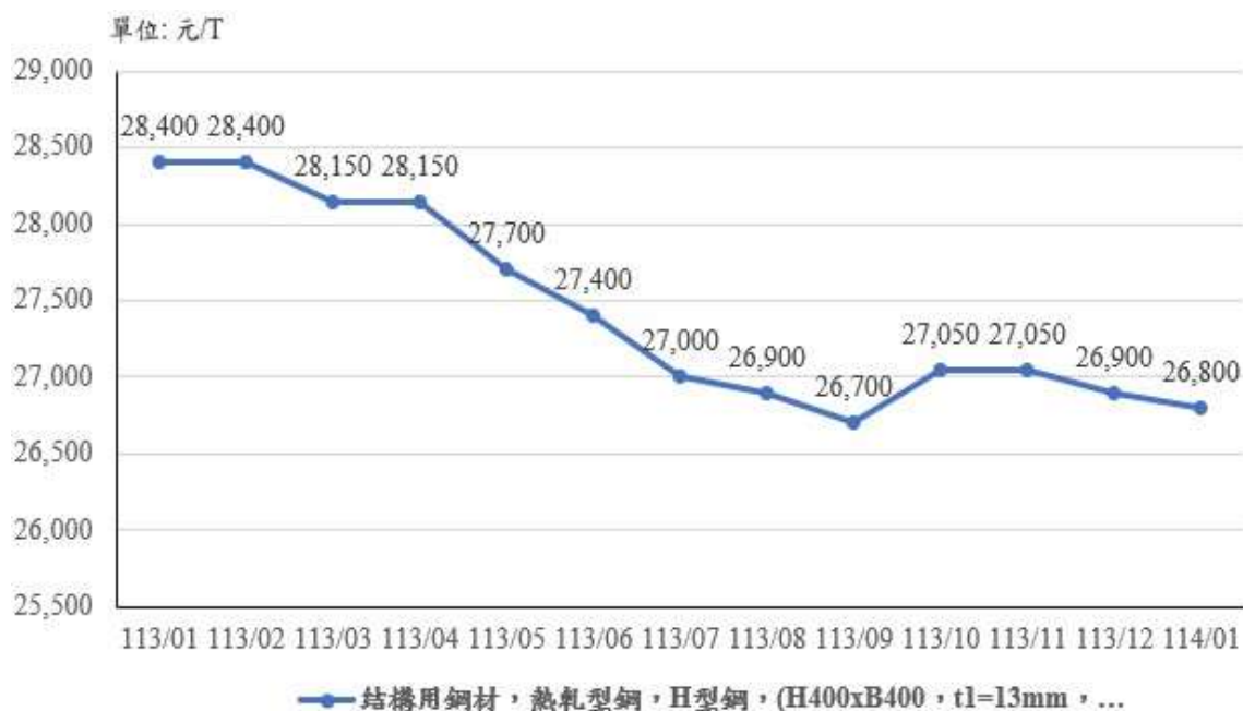
圖 12：113 年 1 月至 114 年 1 月「結構用鋼材，熱軋型鋼，(H400xB400，t1=13mm，t2=21mm)」價格走勢
