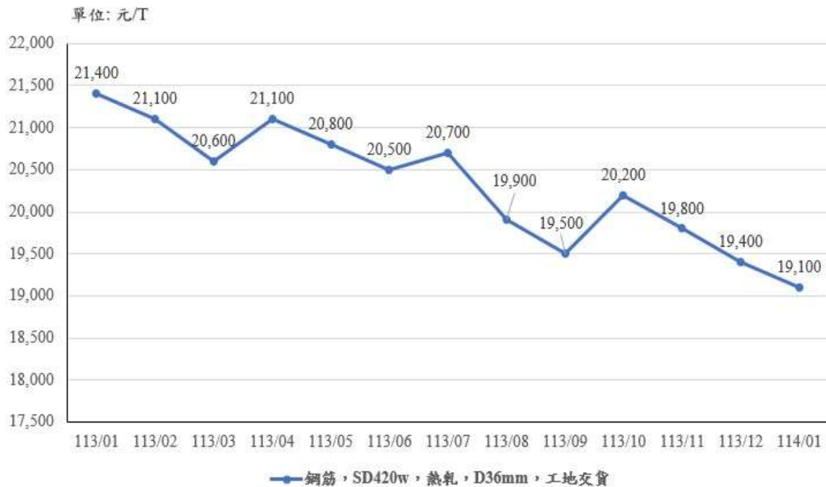
圖 11：113 年 1 月至 114 年 1 月「SD420w，熱軋，D36mm」價格走勢
