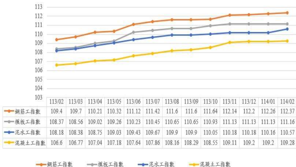
圖 7：113 年 2 月至 114 年 2 月泥水工、鋼筋工、模板工及混凝土工指數走勢
