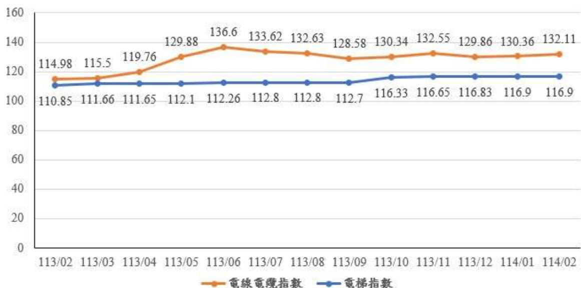
圖 6：113 年 2 月至 114 年 2 月電梯及電線電纜指數走勢
