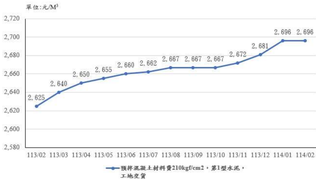
圖 8：113 年 2 月至 114 年 2 月「210kgf/cm 2 ，第 1 型水泥」價格走勢
