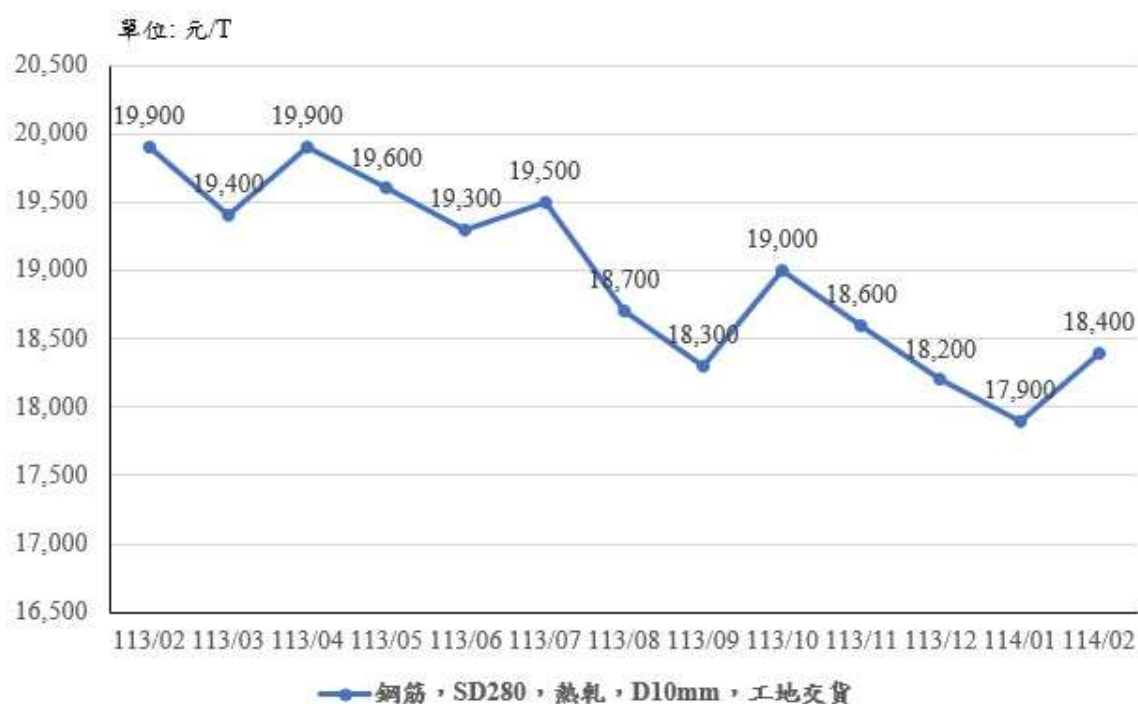
圖 10：：113 年 2 月至 114 年 2 月「SD280，熱軋，D10mm」價格走勢
