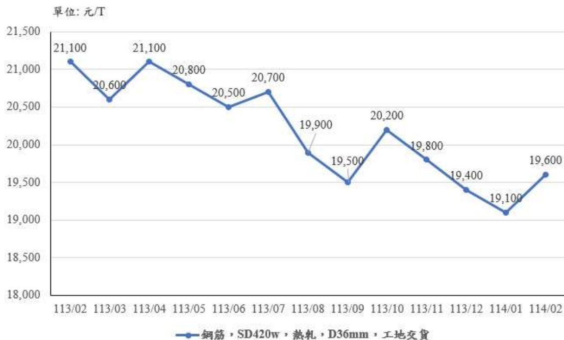
圖 11：113 年 2 月至 114 年 2 月「SD420w，熱軋，D36mm」價格走勢
