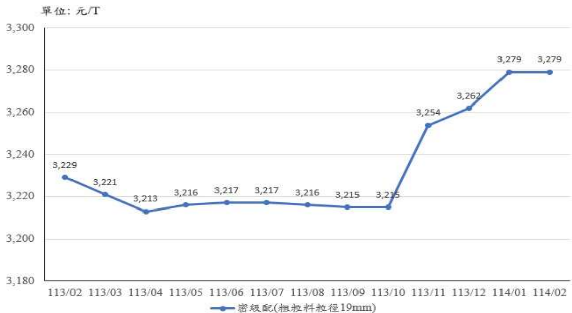
圖 15：113 年 2 月至 114 年 2 月密級配(粗粒料粒徑 19mm)
