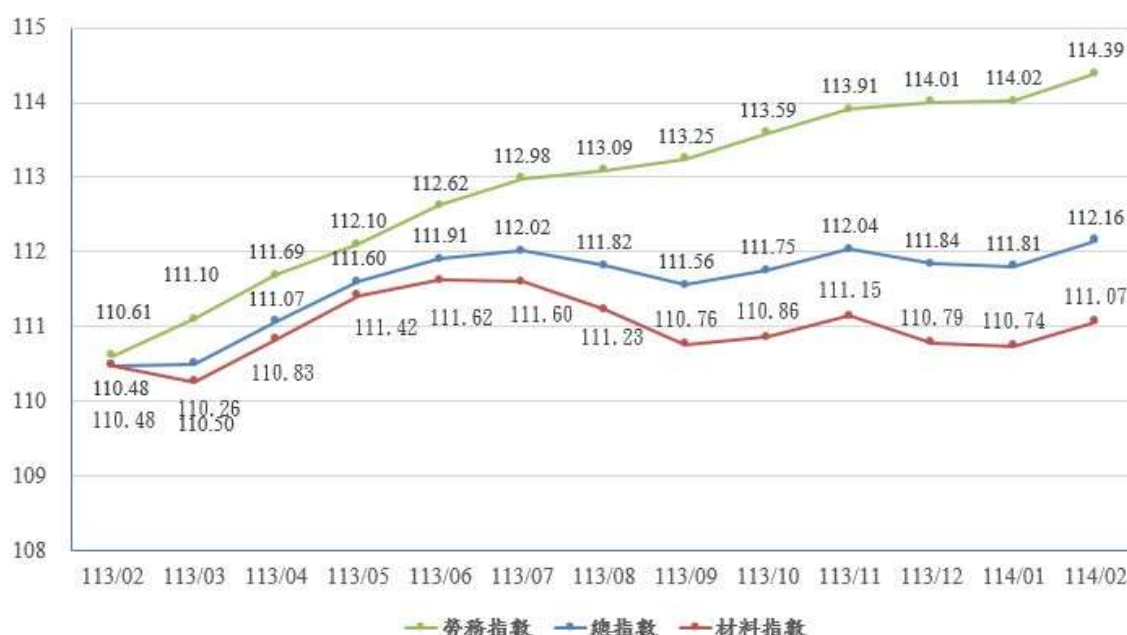
圖 1：113 年 2 月至 114 年 2 月營造工程物價指數走勢。
