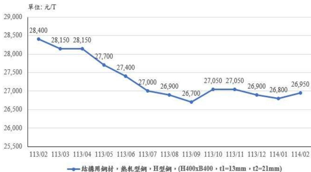
圖 12：113 年 2 月至 114 年 2 月「結構用鋼材，熱軋型鋼，(H400xB400，t1=13mm，t2=21mm)」價格走勢
