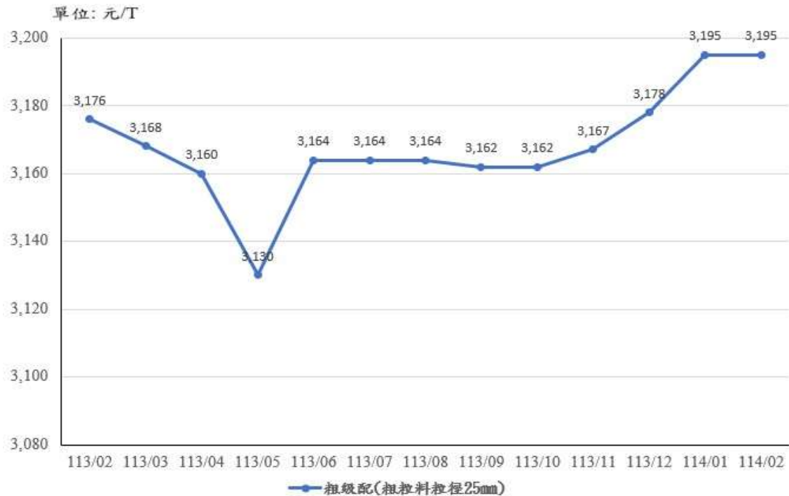
圖 14：113 年 2 月至 114 年 2 月粗級配(粗粒料粒徑 25mm)
