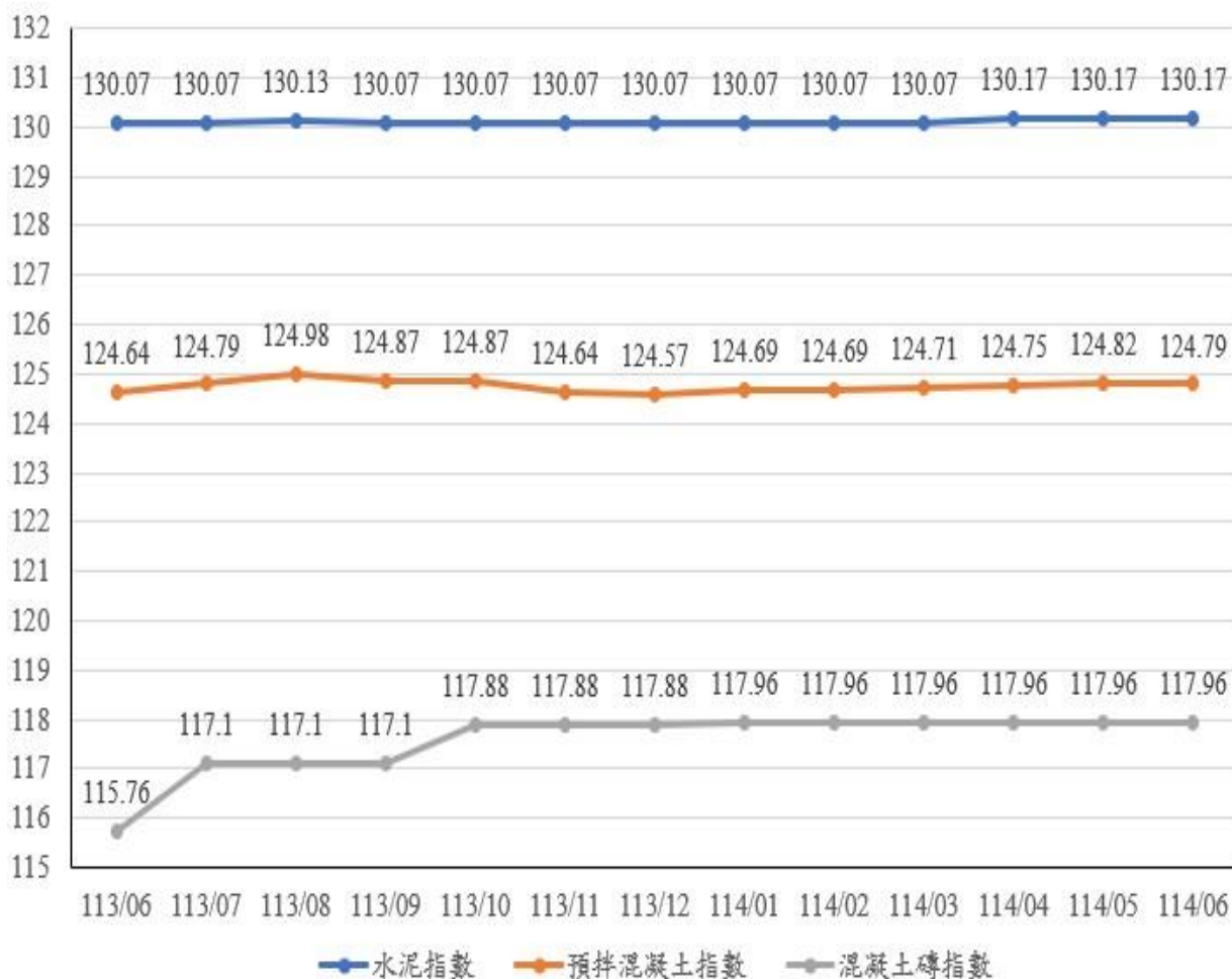
圖 2：113 年 6 月至 114 年 6 月水泥、預拌混凝土及混凝土磚指數走勢
