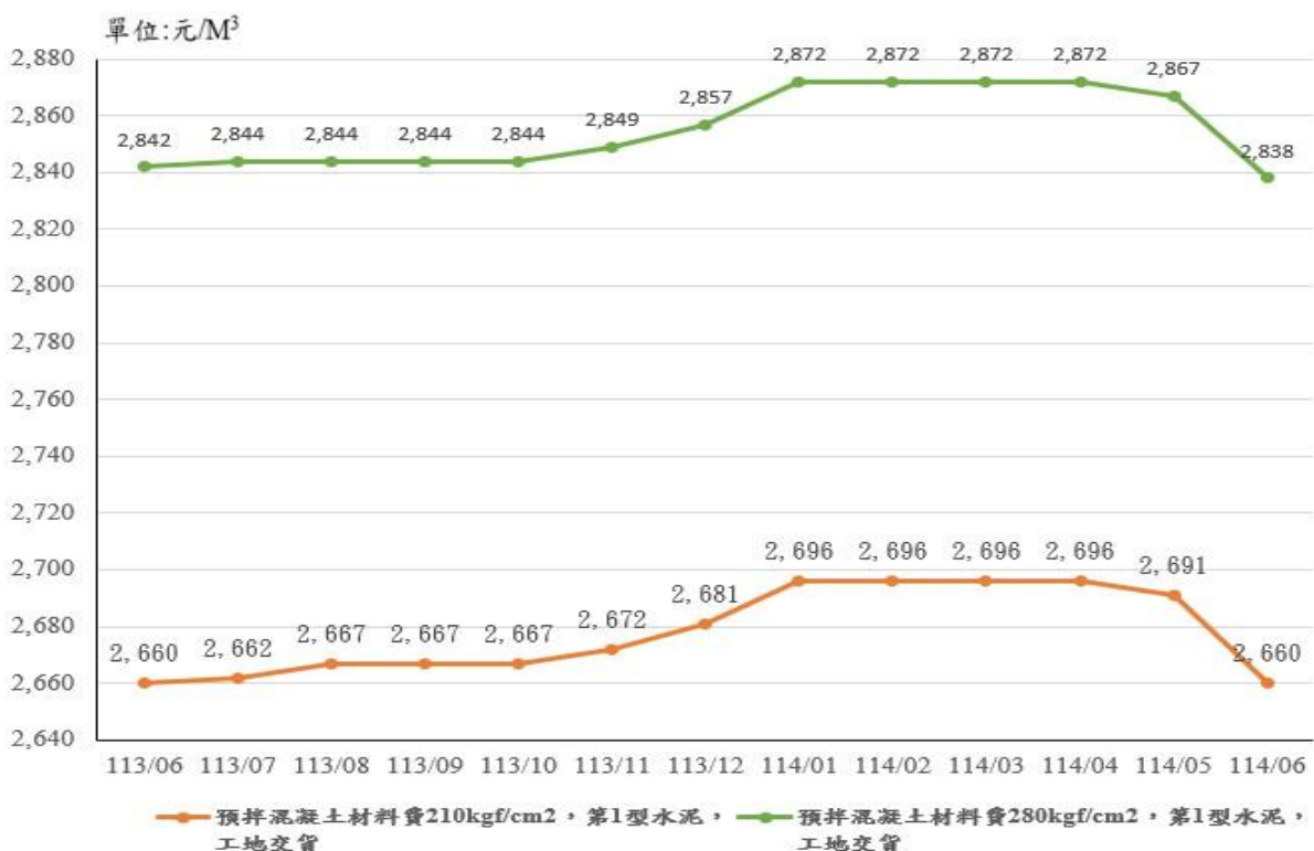
圖 8：113 年 6 月至 114 年 6 月「第 1 型水泥-210kgf/cm 2 及 280kgf/cm 2 」價格走勢
