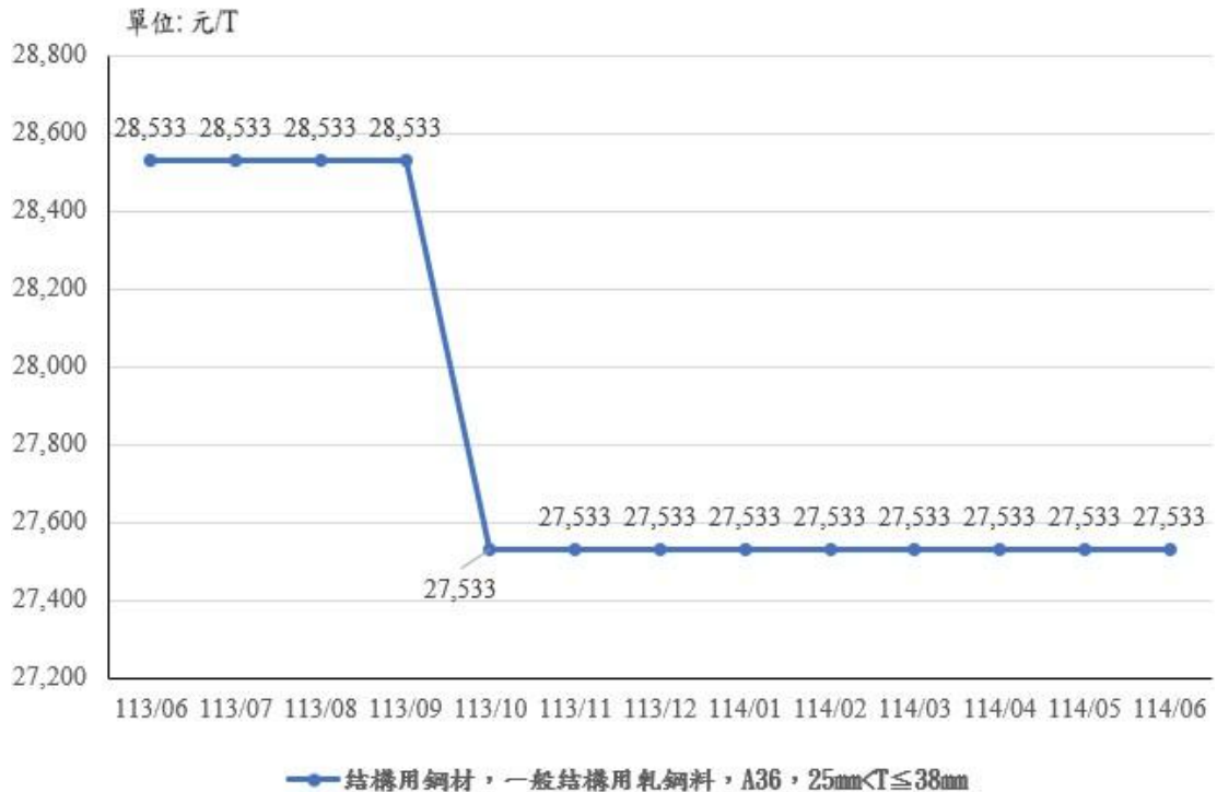
圖 11：113 年 6 月至 114 年 6 月「結構用鋼材，一般結構用軋鋼料，A36，25mm<T≤38mm」價格走勢
