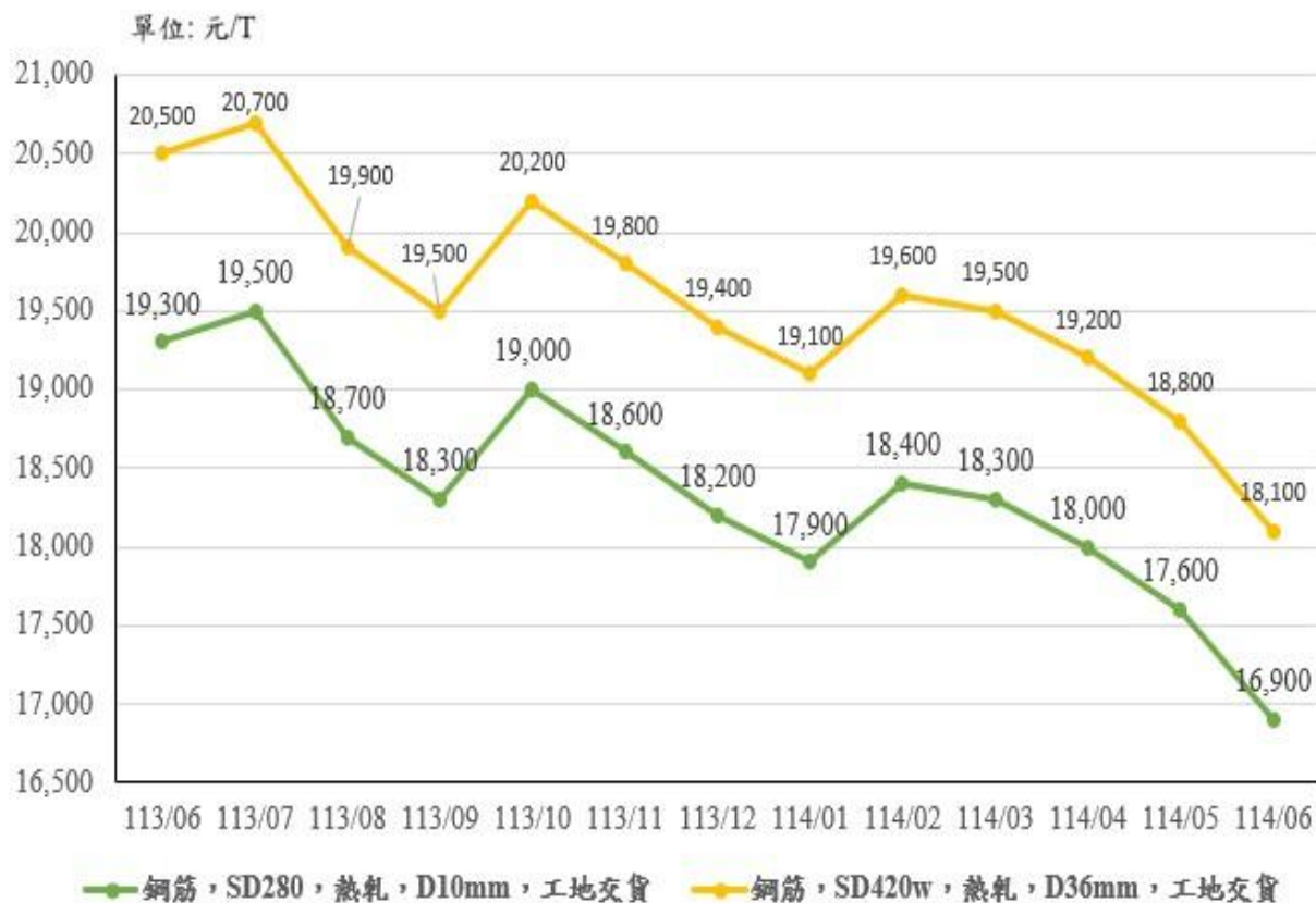
圖 9：：113 年 6 月至 114 年 6 月「SD280，熱軋，D10mm；SD420w，熱軋，D36mm」價格走勢
