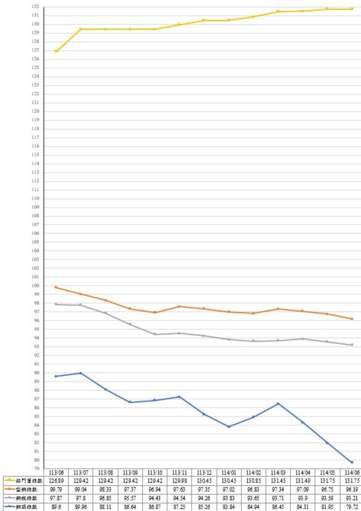
圖 4：113 年 6 月至 114 年 6 月鋁門窗、型鋼、鋼板及鋼筋指數走勢
