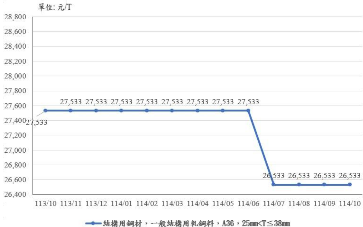
圖 11：113 年 10 月至 114 年 10 月「結構用鋼材，一般結構用軋鋼料，A36，25mm<T≤38mm」價格走勢
