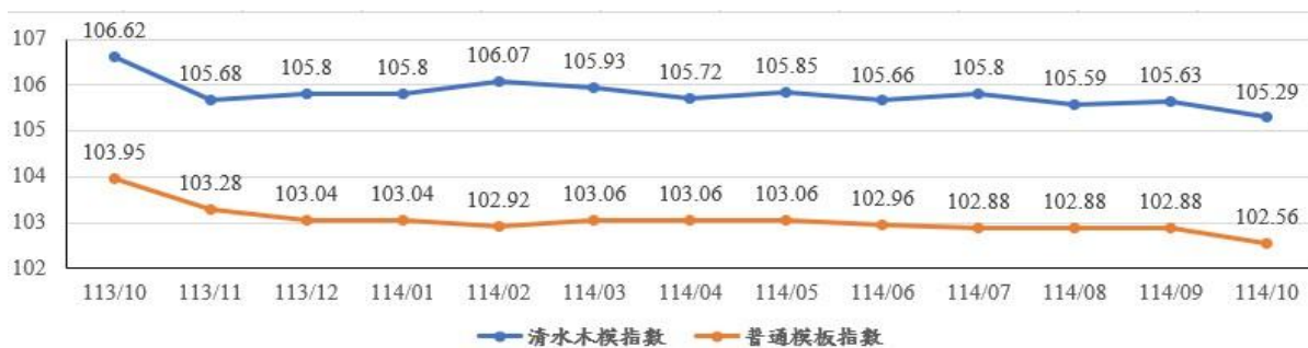
圖 5：113 年 10 月至 114 年 10 月清水木模及普通模板指數走勢
