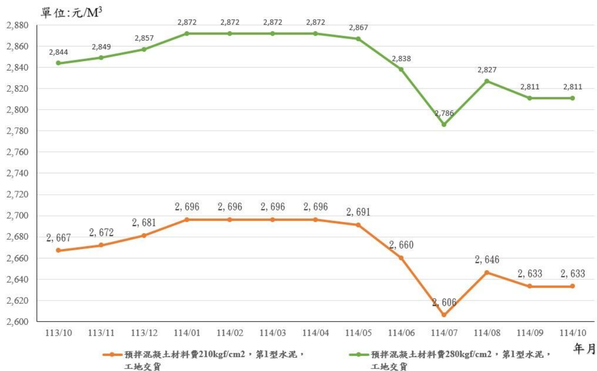
圖 8：113 年 10 月至 114 年 10 月「第 1 型水泥-210kgf/cm 2 及 280kgf/cm 2 」價格走勢
