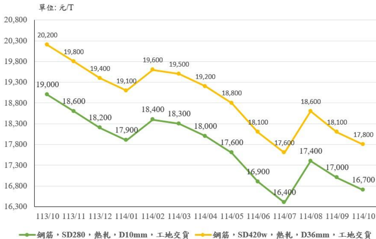
圖 9：：113 年 10 月至 114 年 10 月「SD280，熱軋，D10mm；SD420w，熱軋，D36mm」價格走勢
