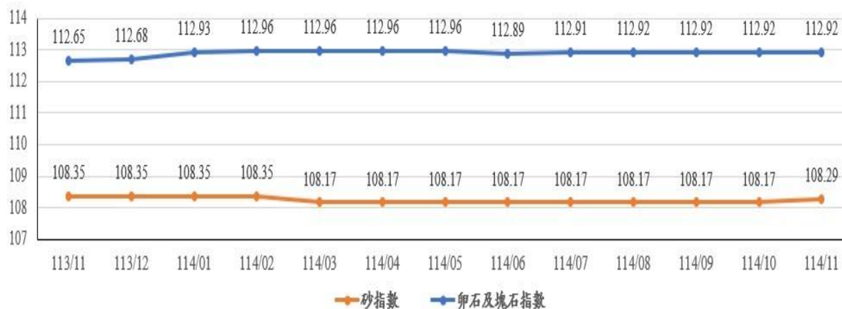
圖 3：113 年 11 月至 114 年 11 月砂、卵石及塊石指數走勢
