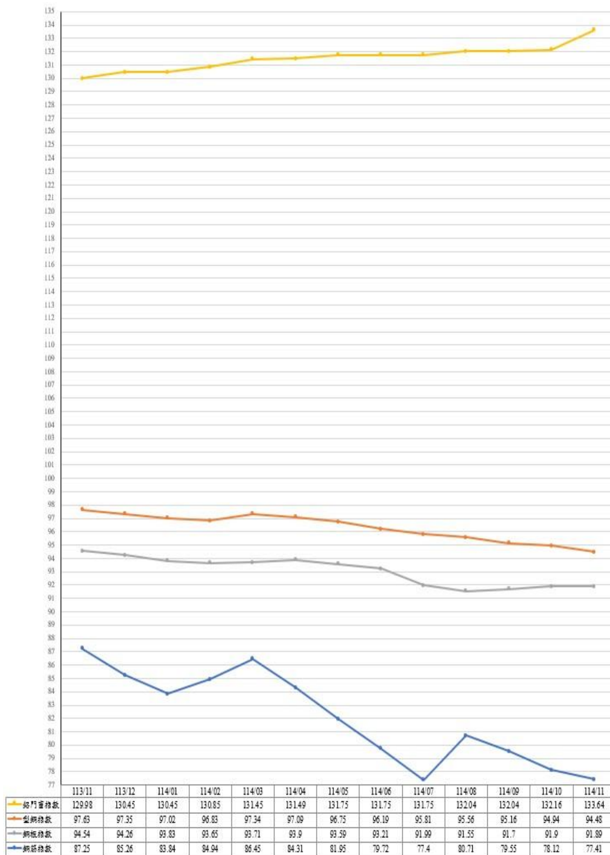
圖 4：113 年 11 月至 114 年 11 月鋁門窗、型鋼、鋼板及鋼筋指數走勢
