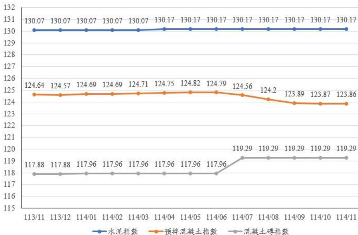
圖 2：113 年 11 月至 114 年 11 月水泥、預拌混凝土及混凝土磚指數走勢
