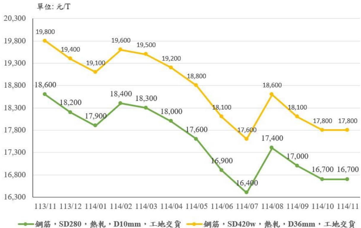
圖 9：：113 年 11 月至 114 年 11 月「SD280，熱軋，D10mm；SD420w，熱軋，D36mm」價格走勢
