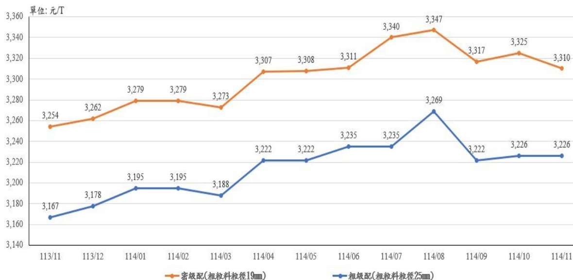
圖 12：113 年 11 月至 114 年 11 月「密級配(粗粒料粒徑 19mm)及粗級配(粗粒料粒徑 25mm)」價格走勢
