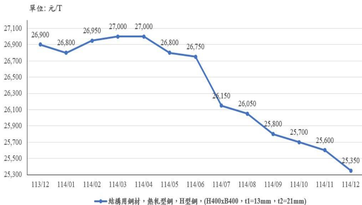
圖 10：113 年 12 月至 114 年 12 月「結構用鋼材，熱軋型鋼，(H400xB400，t1=13mm，t2=21mm)」價格走勢
