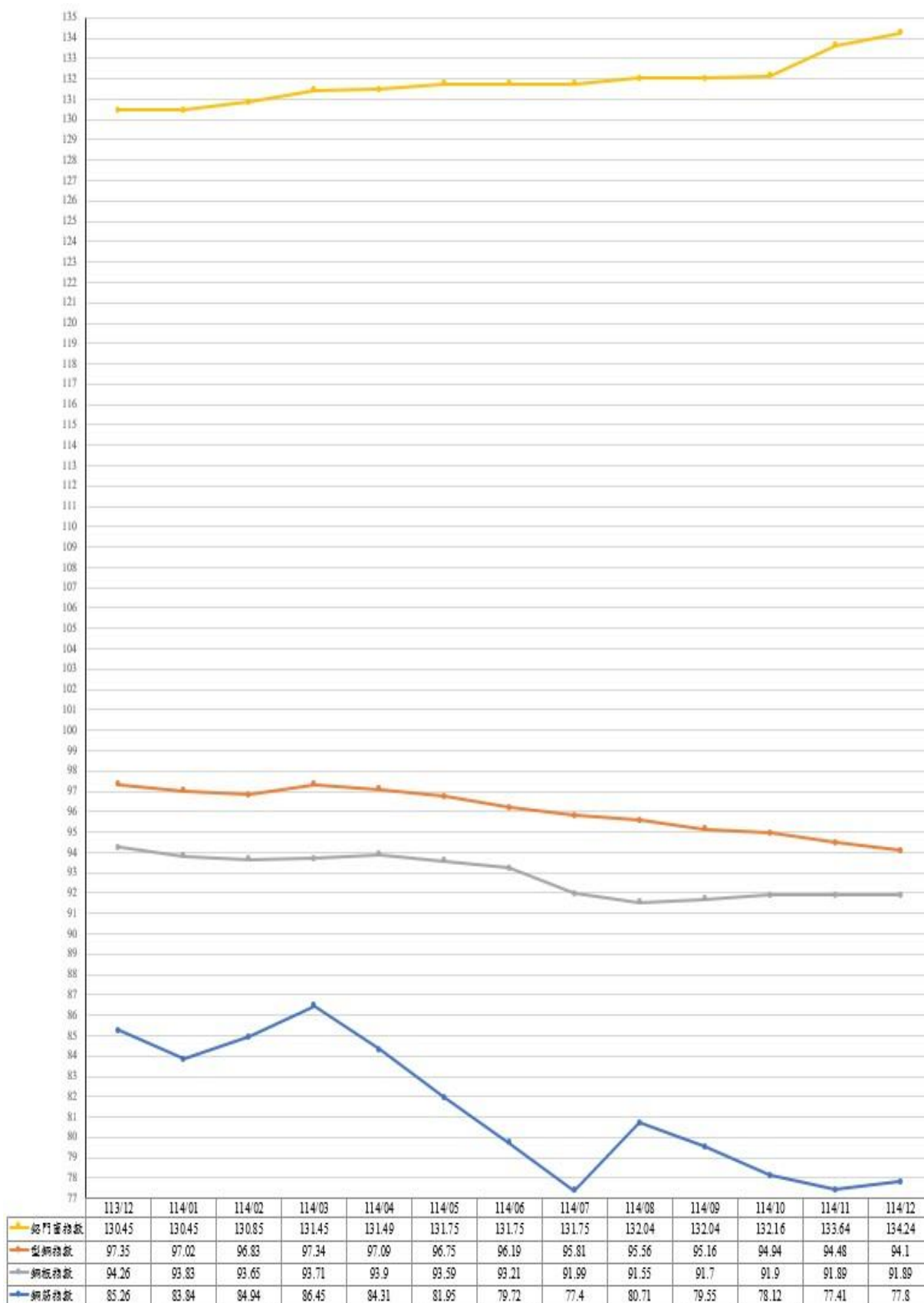
圖 4：113 年 12 月至 114 年 12 月鋁門窗、型鋼、鋼板及鋼筋指數走勢
