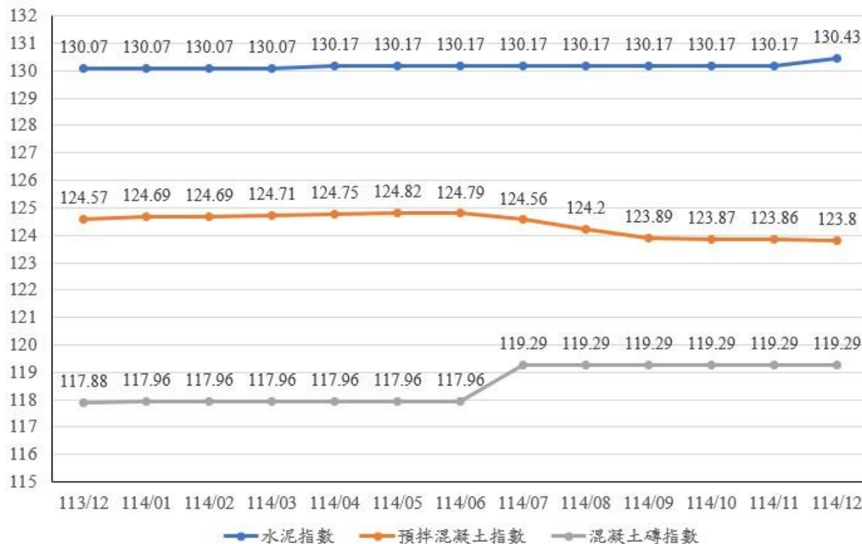
圖 2：113 年 12 月至 114 年 12 月水泥、預拌混凝土及混凝土磚指數走勢
