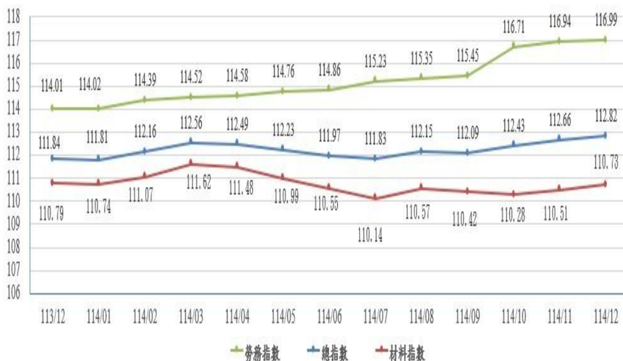
圖 1：113 年 12 月至 114 年 12 月營造工程物價指數走勢。
