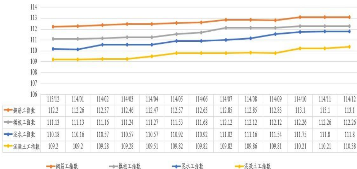
圖 7：113 年 12 月至 114 年 12 月鋼筋工、模板工、泥水工及混凝土工指數走勢
