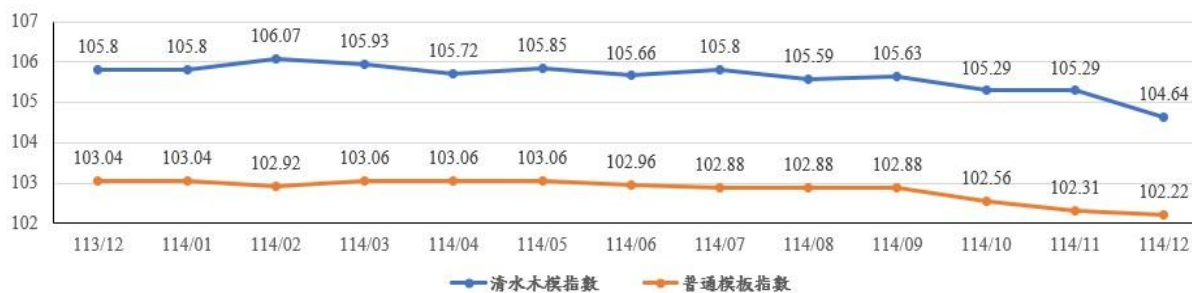
圖 5：113 年 12 月至 114 年 12 月清水木模及普通模板指數走勢
