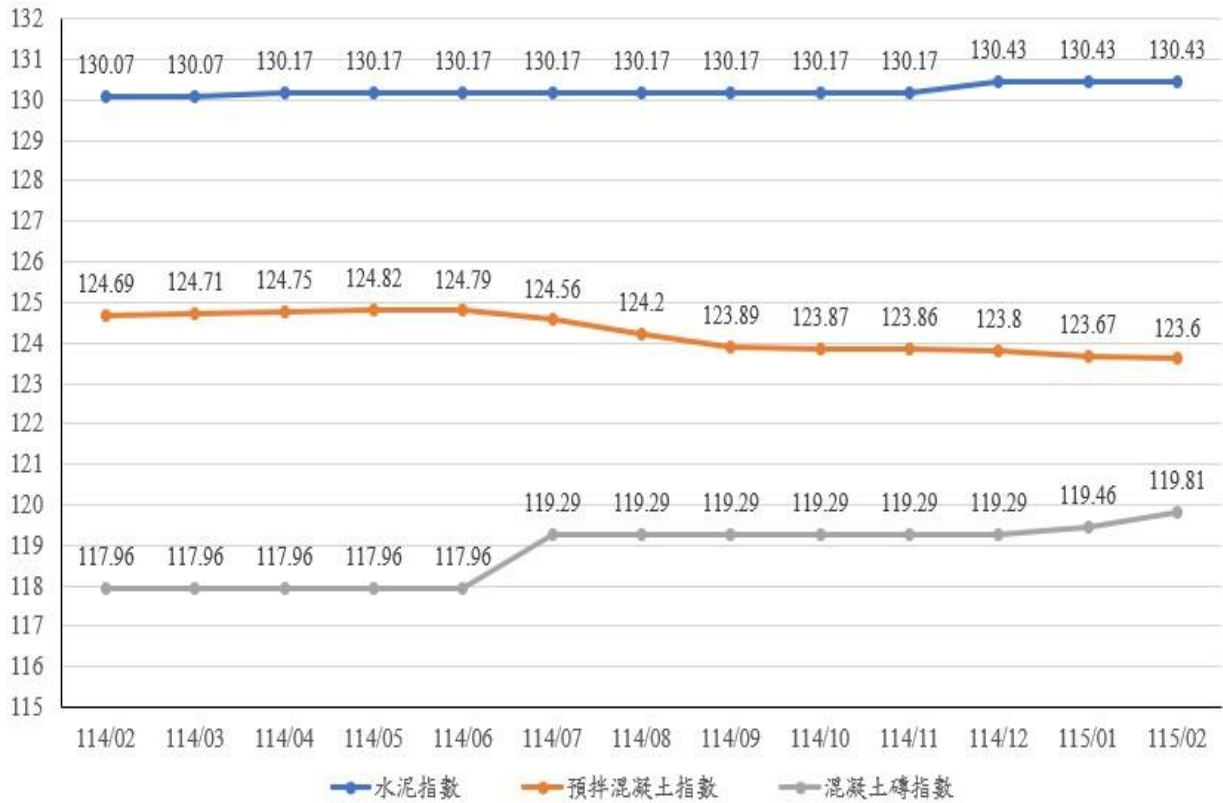
圖 2：114 年 2 月至 115 年 2 月水泥、預拌混凝土及混凝土磚指數走勢
