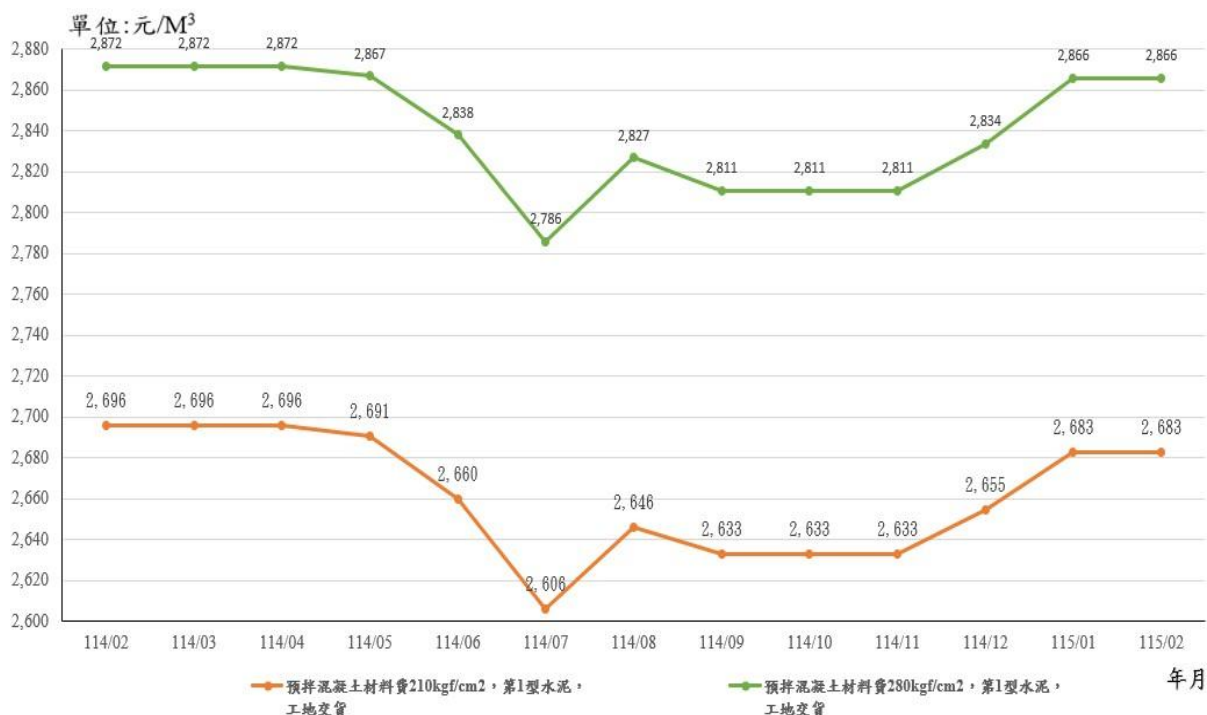
圖 8：114 年 2 月至 115 年 2 月「第 1 型水泥-210kgf/cm 2 及 280kgf/cm 2 」價格走勢
