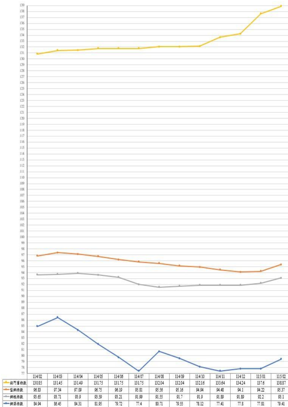
圖 4：114 年 2 月至 115 年 2 月鋁門窗、型鋼、鋼板及鋼筋指數走勢
