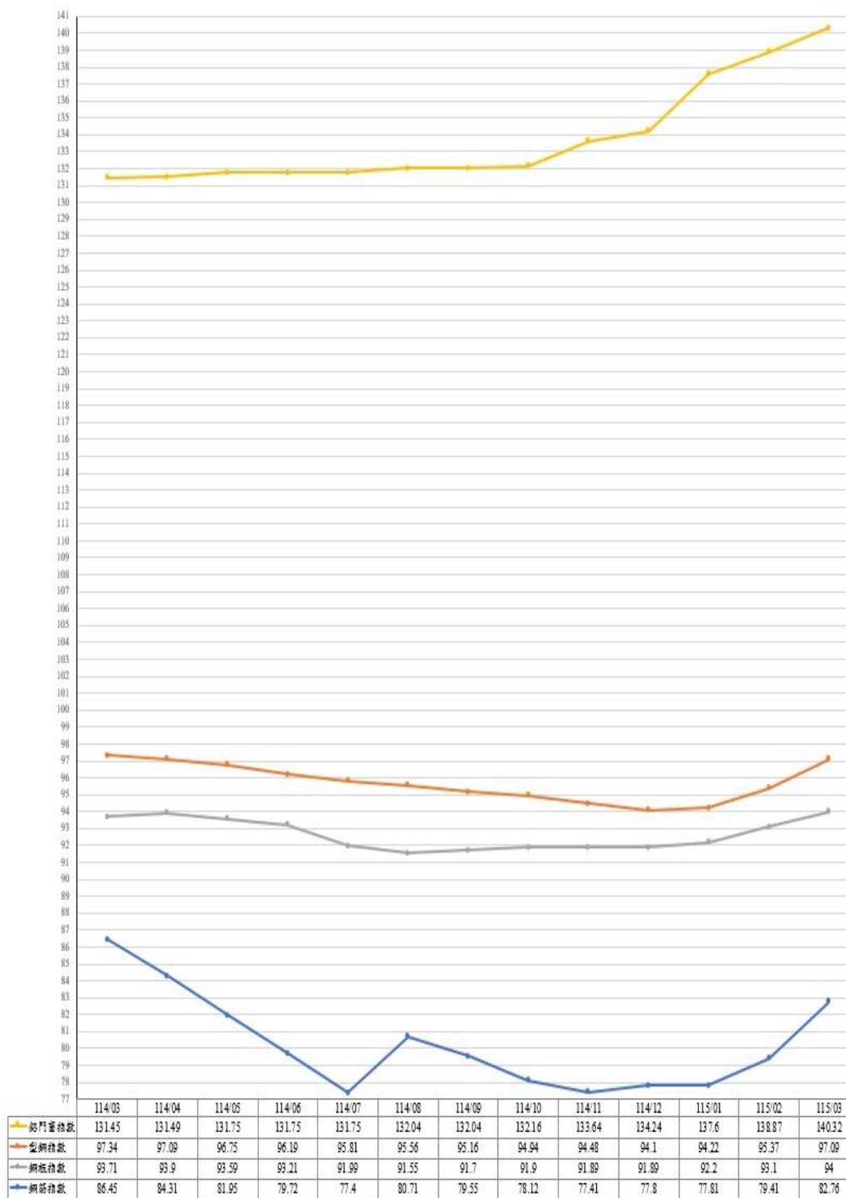
圖 4：114 年 3 月至 115 年 3 月鋁門窗、型鋼、鋼板及鋼筋指數走勢
