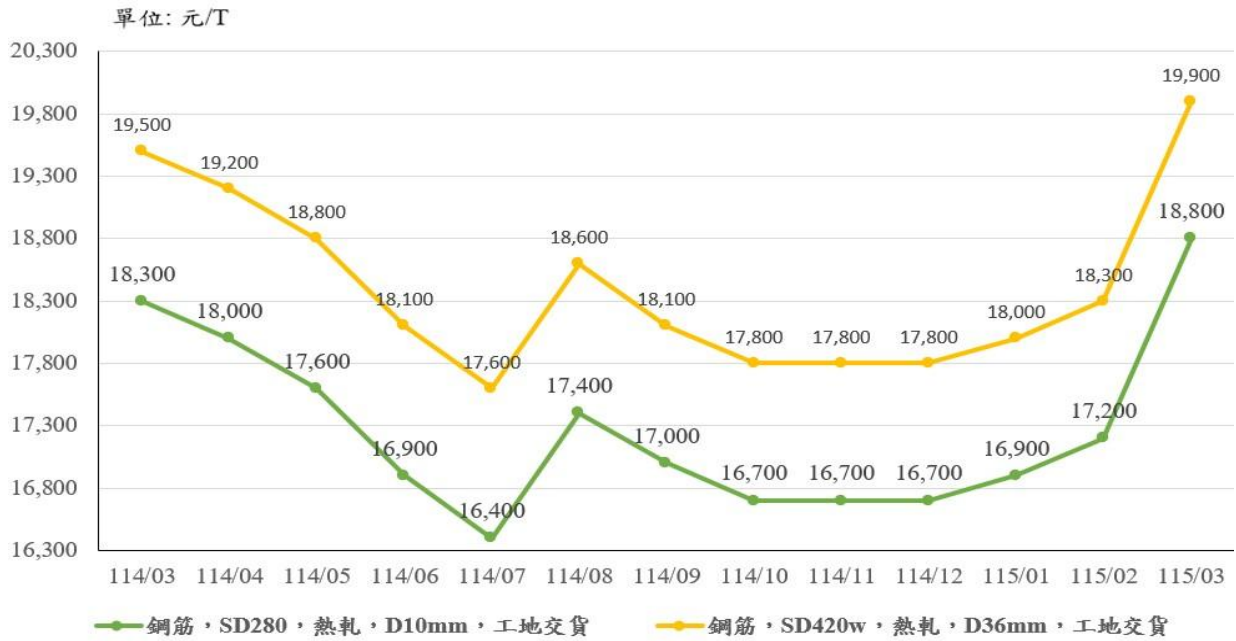
圖 9：：114 年 3 月至 115 年 3 月「SD280，熱軋，D10mm；SD420w，熱軋，D36mm」價格走勢
