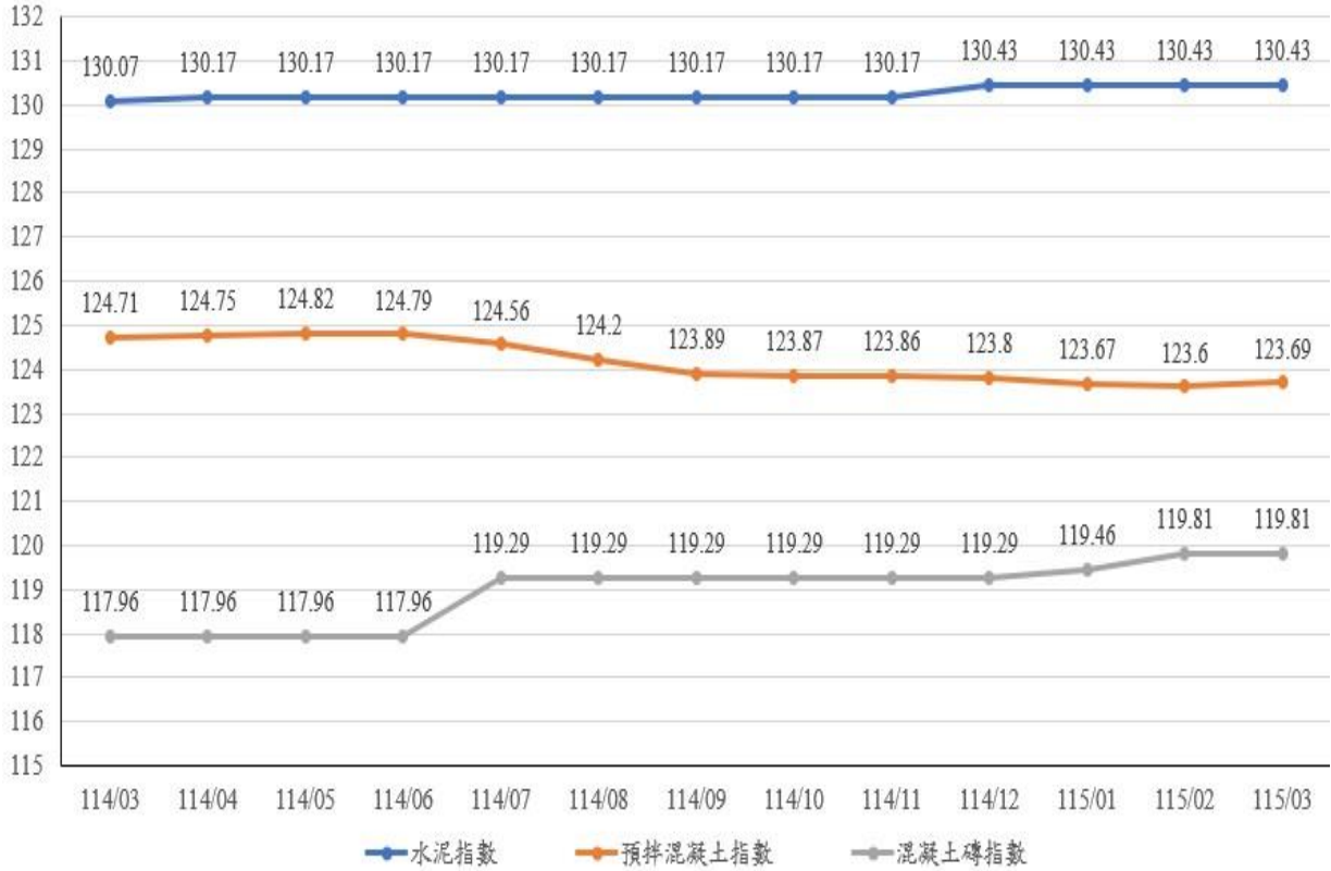
圖 2：114 年 3 月至 115 年 3 月水泥、預拌混凝土及混凝土磚指數走勢
