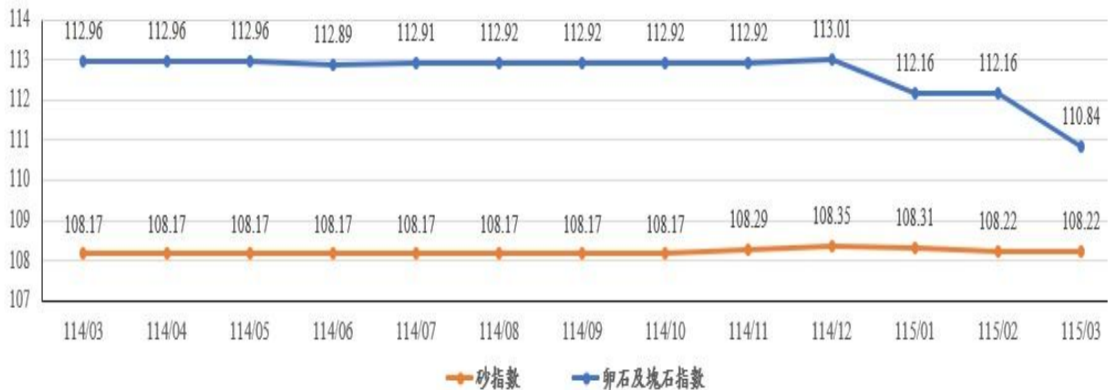
圖 3：114 年 3 月至 115 年 3 月砂、卵石及塊石指數走勢
