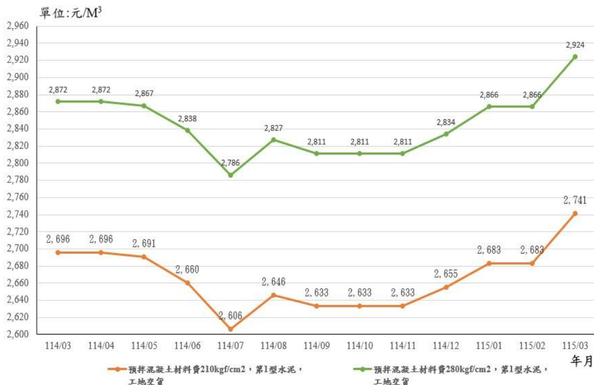
圖 8：114 年 3 月至 115 年 3 月「第 1 型水泥-210kgf/cm 2 及 280kgf/cm 2 」價格走勢
