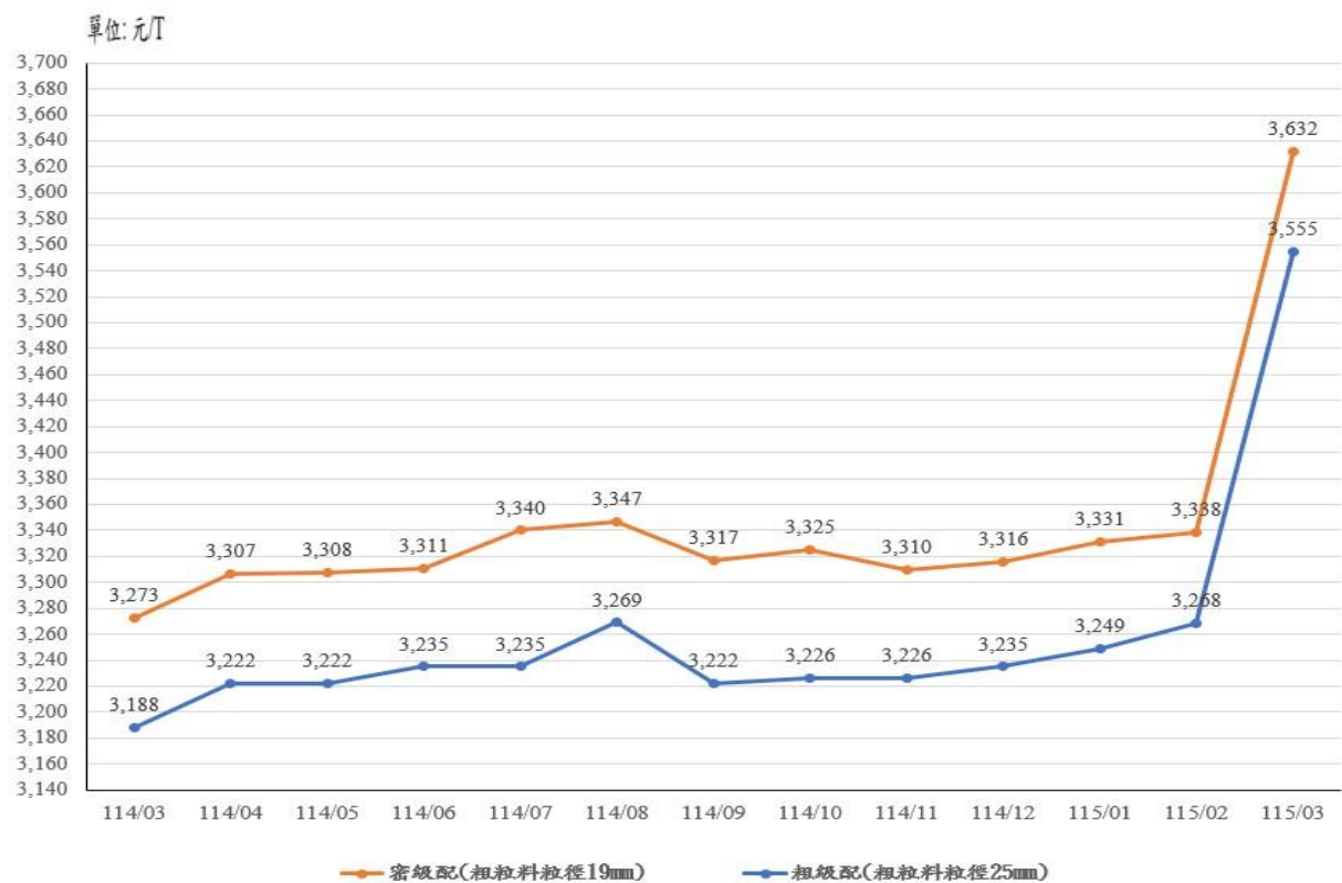
圖 12：114 年 3 月至 115 年 3 月「密級配(粗粒料粒徑 19mm)及粗級配(粗粒料粒徑 25mm)」價格走勢
