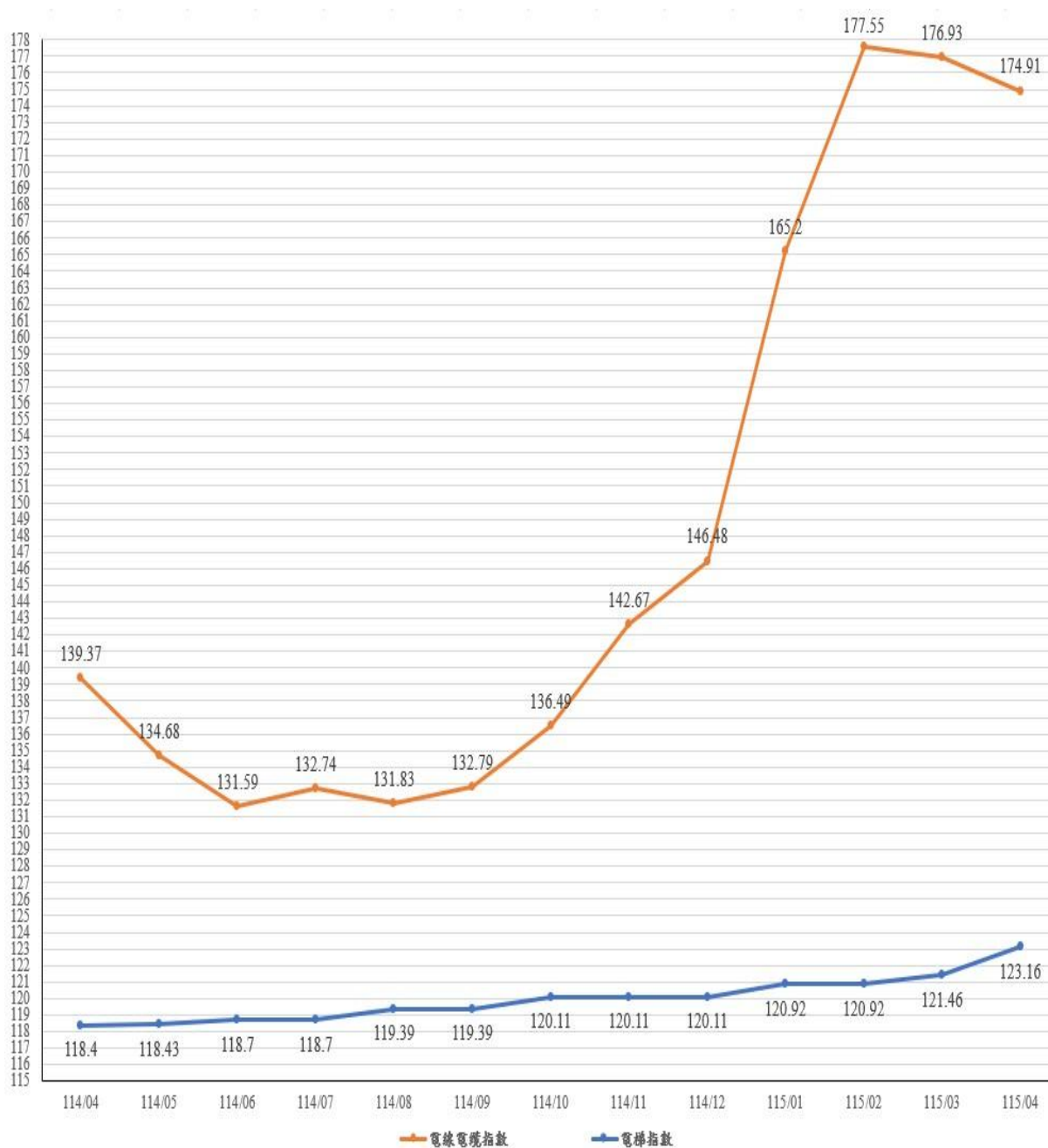
圖 6：114 年 4 月至 115 年 4 月電線電纜及電梯指數走勢
