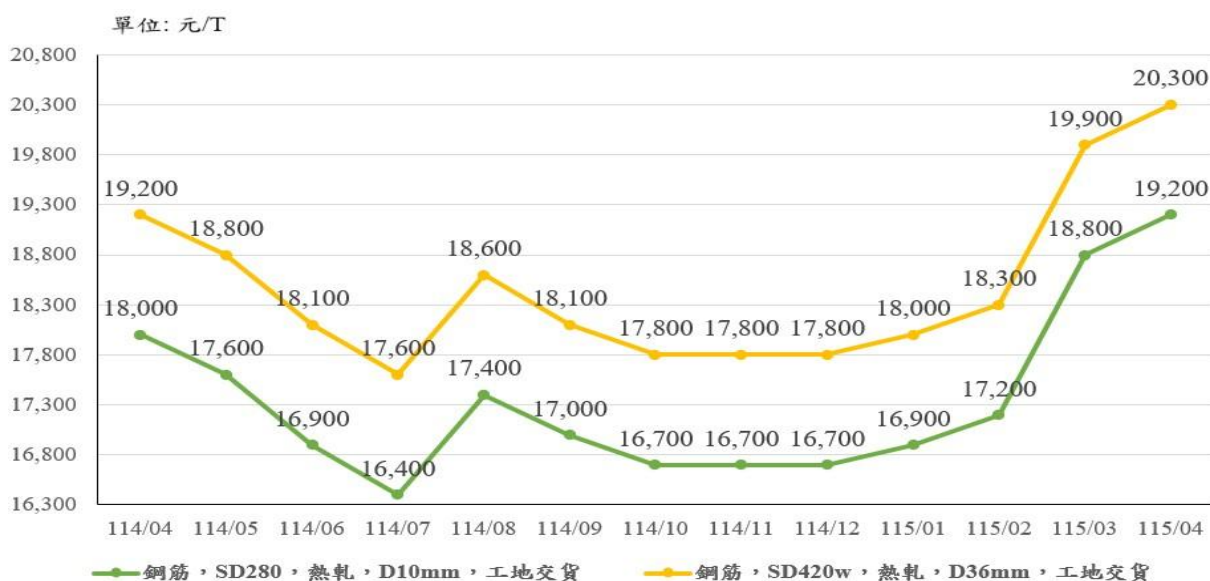
圖 10：：114 年 4 月至 115 年 4 月「SD280，熱軋，D10mm；SD420w，熱軋，D36mm」價格走勢
