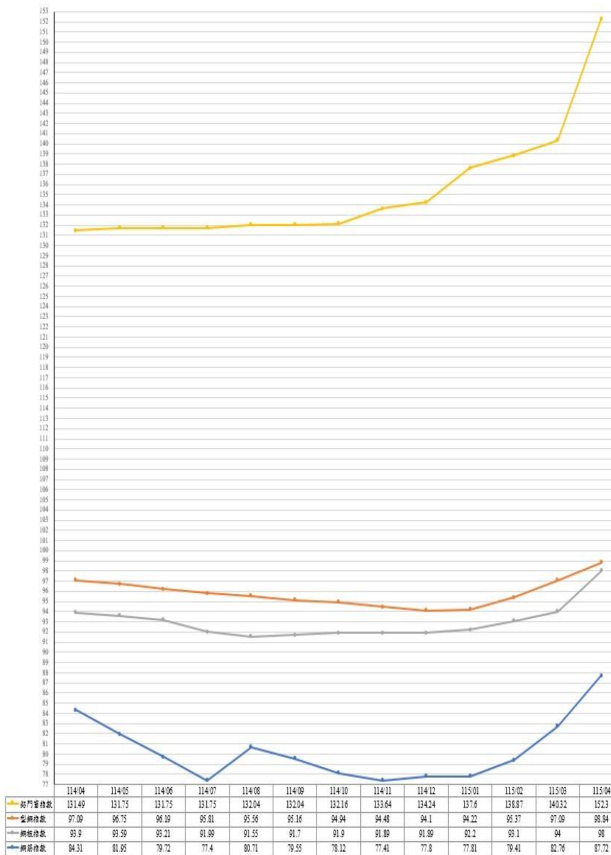
圖 4：114 年 4 月至 115 年 4 月鋁門窗、型鋼、鋼板及鋼筋指數走勢
