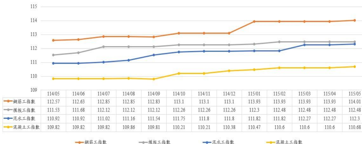
圖 7：114 年 5 月至 115 年 5 月鋼筋工、模板工、泥水工及混凝土工指數走勢
