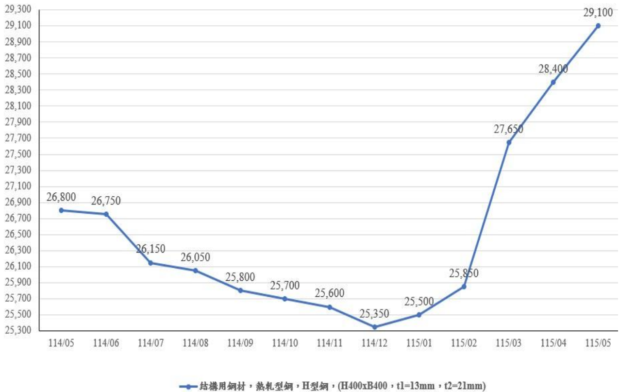
圖 11：114 年 5 月至 115 年 5 月「結構用鋼材，熱軋型鋼，(H400xB400，t1=13mm，t2=21mm)」價格走勢
