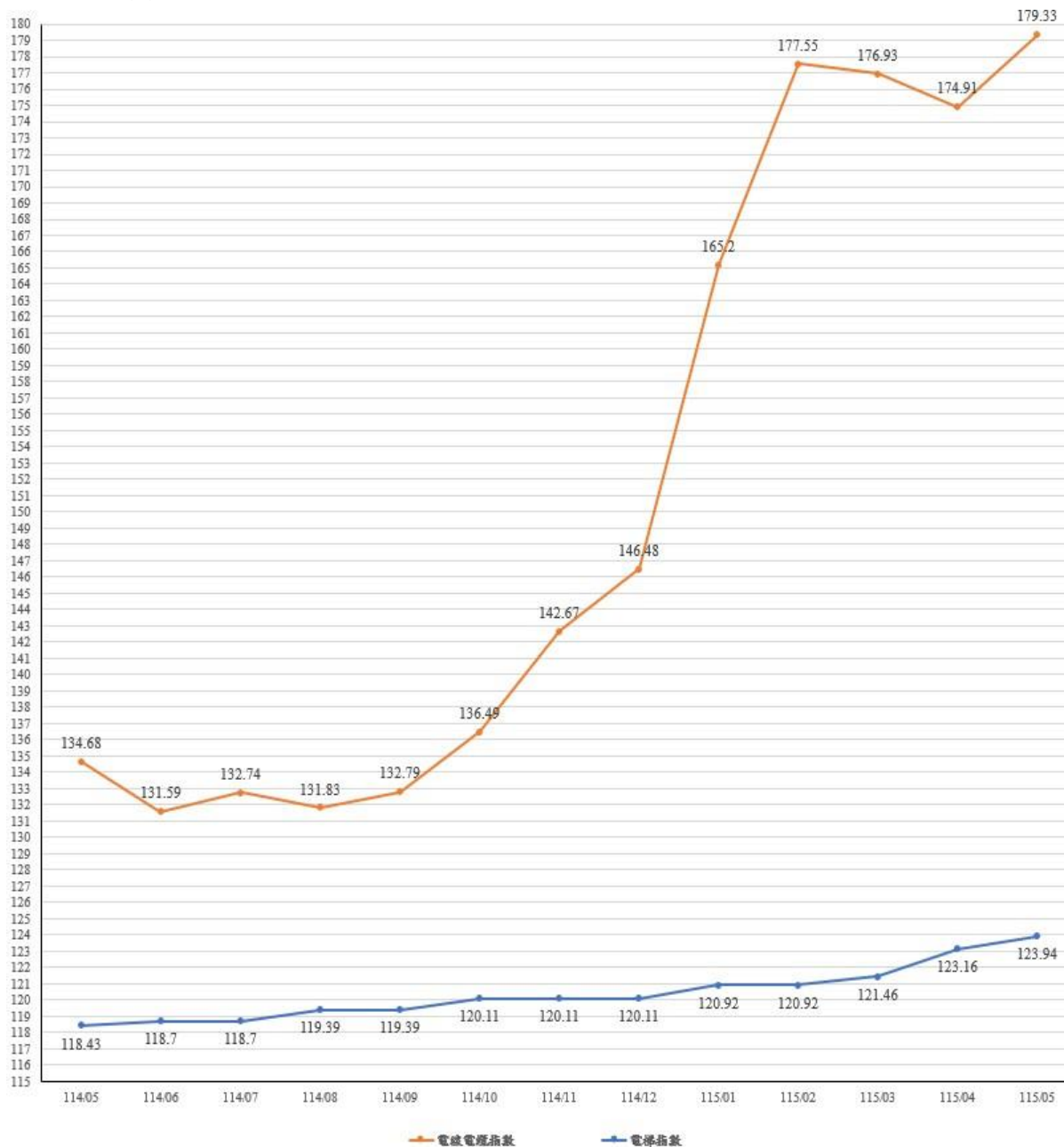
圖 6：114 年 5 月至 115 年 5 月電線電纜及電梯指數走勢
