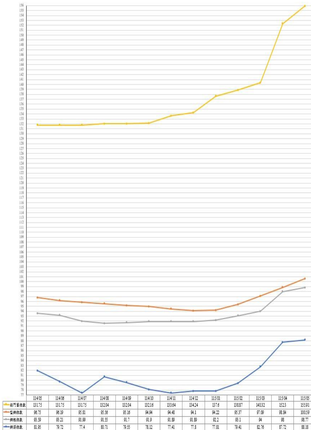
圖 4：114 年 5 月至 115 年 5 月鋁門窗、型鋼、鋼板及鋼筋指數走勢
