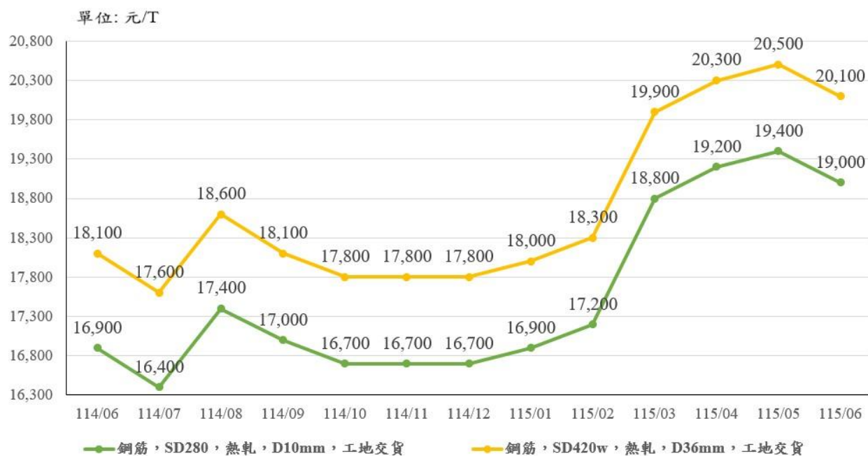
圖 10：：114 年 6 月至 115 年 6 月「SD280，熱軋，D10mm；SD420w，熱軋，D36mm」價格走勢
