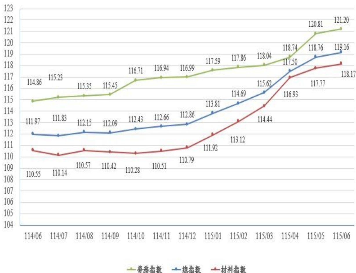
圖 1：114 年 6 月至 115 年 6 月營造工程物價指數走勢。
