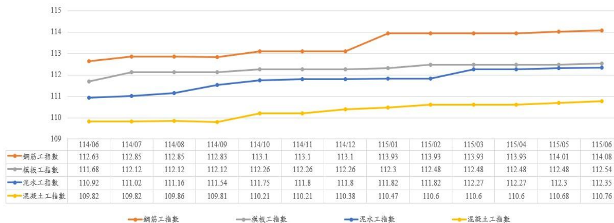
圖 7：114 年 6 月至 115 年 6 月鋼筋工、模板工、泥水工及混凝土工指數走勢
