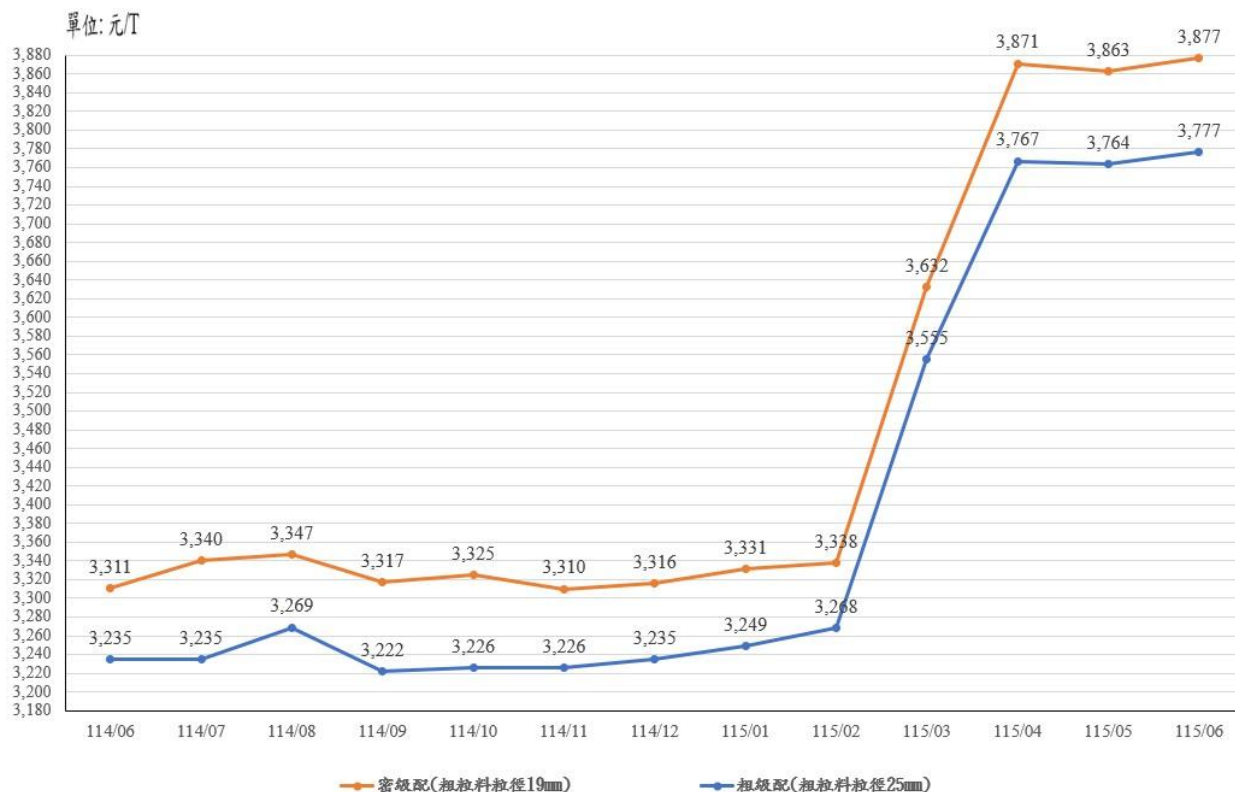
圖 9：114 年 6 月至 115 年 6 月「密級配(粗粒料粒徑 19mm)及粗級配(粗粒料粒徑 25mm)」價格走勢
