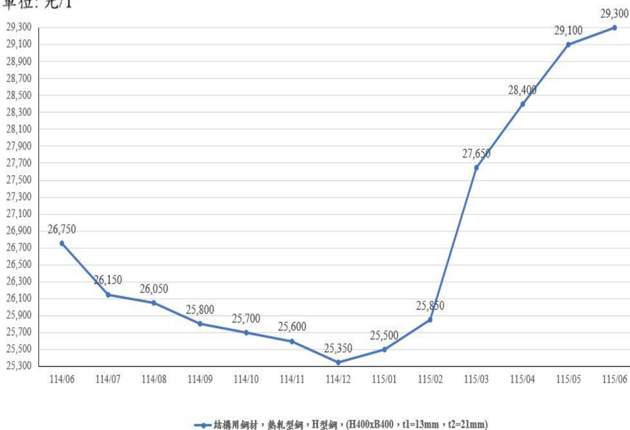
圖 11：114 年 6 月至 115 年 6 月「結構用鋼材，熱軋型鋼，(H400xB400，t1=13mm，t2=21mm)」
