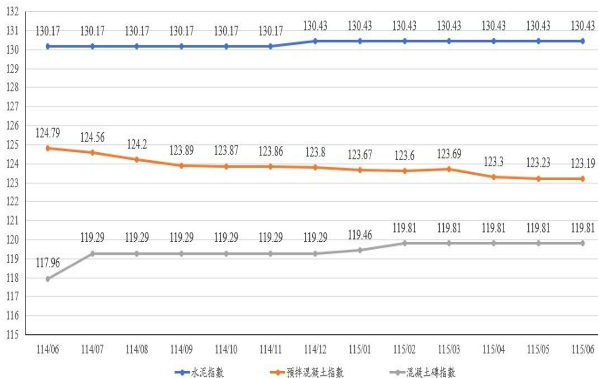
圖 2：114 年 6 月至 115 年 6 月水泥、預拌混凝土及混凝土磚指數走勢
