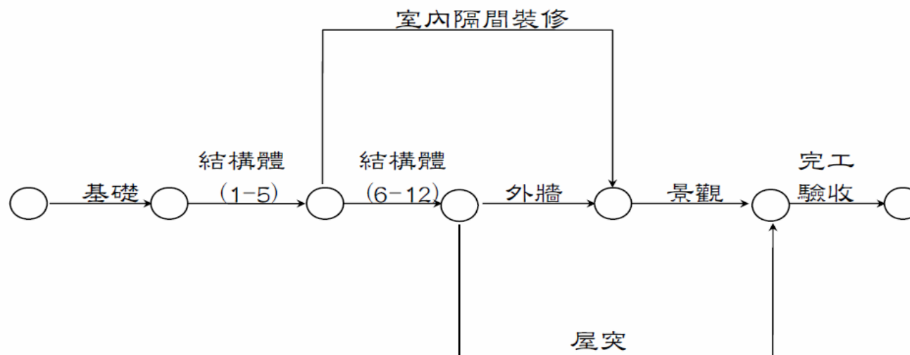
進度網圖要徑（簡例/非完整）
