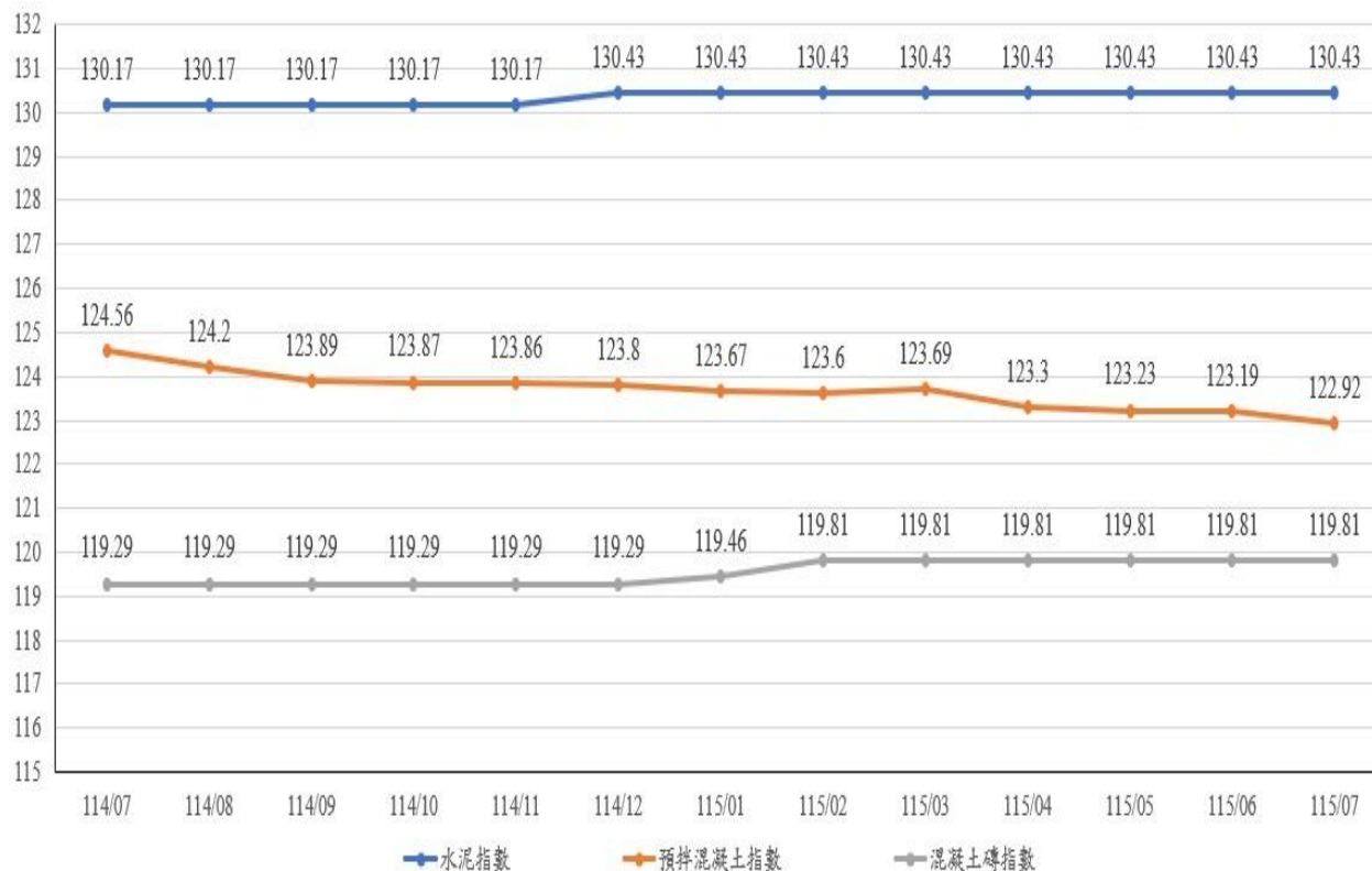
圖 2：114 年 7 月至 115 年 7 月水泥、預拌混凝土及混凝土磚指數走勢
