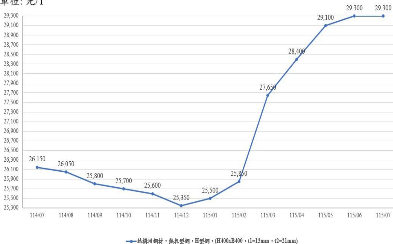
圖 11：114 年 7 月至 115 年 7 月「結構用鋼材，熱軋型鋼，(H400xB400，t1=13mm，t2=21mm)」價格走勢
