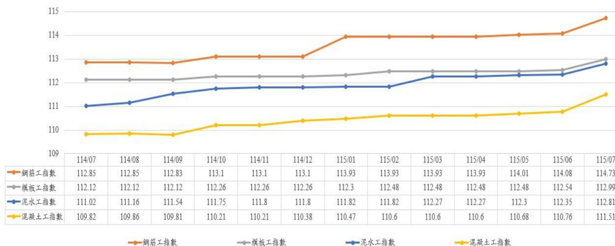
圖 7：114 年 7 月至 115 年 7 月鋼筋工、模板工、泥水工及混凝土工指數走勢
