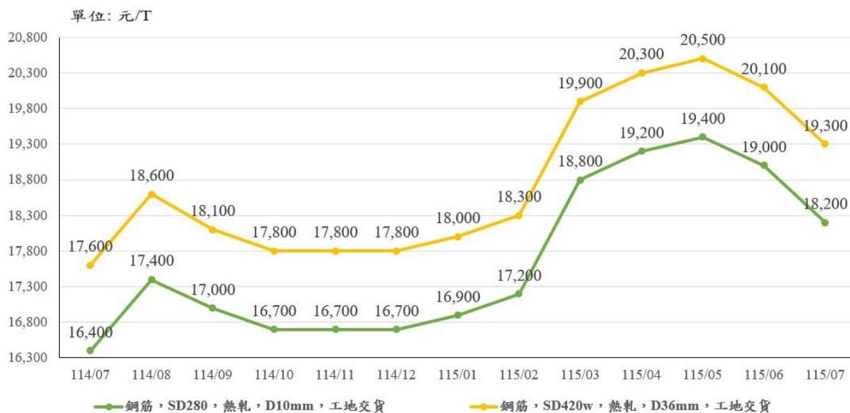
圖 10：：114 年 7 月至 115 年 7 月「SD280，熱軋，D10mm；SD420w，熱軋，D36mm」價格走勢
