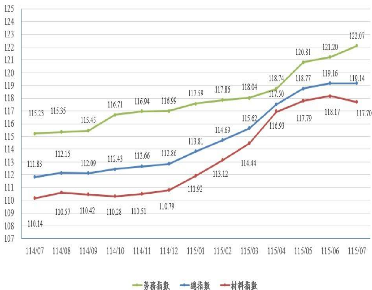
圖 1：114 年 7 月至 115 年 7 月營造工程物價指數走勢。
