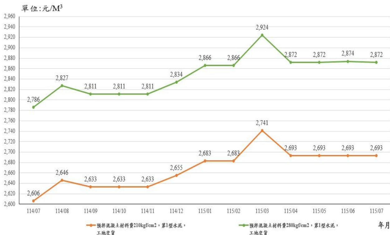
圖 8：114 年 7 月至 115 年 7 月「第 1 型水泥-210kgf/cm 2 及 280kgf/cm 2 」價格走勢
